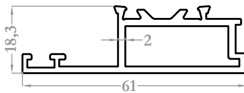
2624 0,696 kg/m
