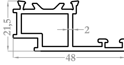
2603 0,661 kg/m
