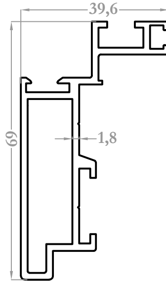
3503 1,005 kg/m
