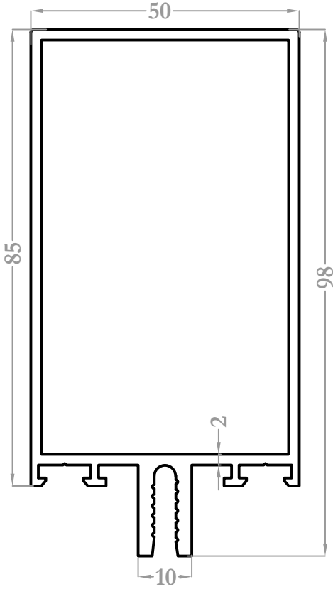
3214 1,730 kg/m
