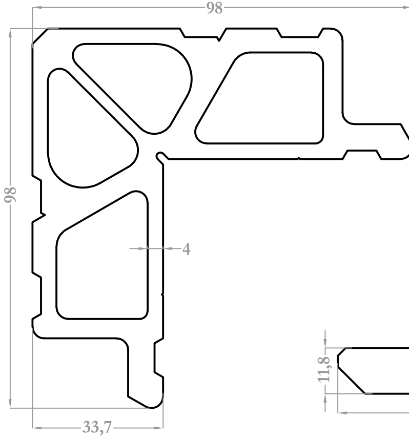
3054 5,840 kg/m
