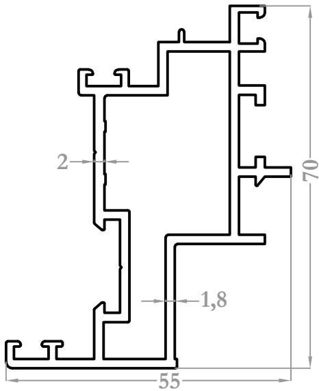
3502 1,305 kg/m
