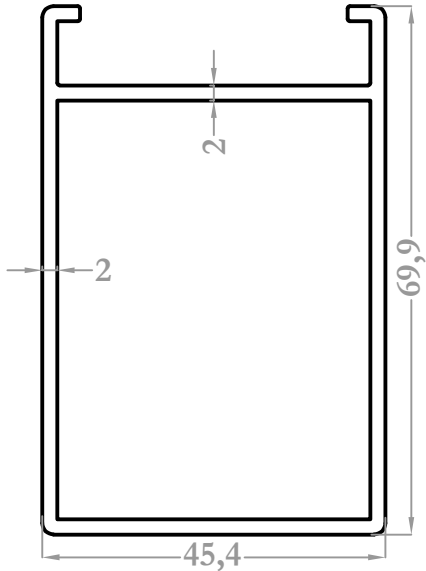
8603 1,233 kg/m
