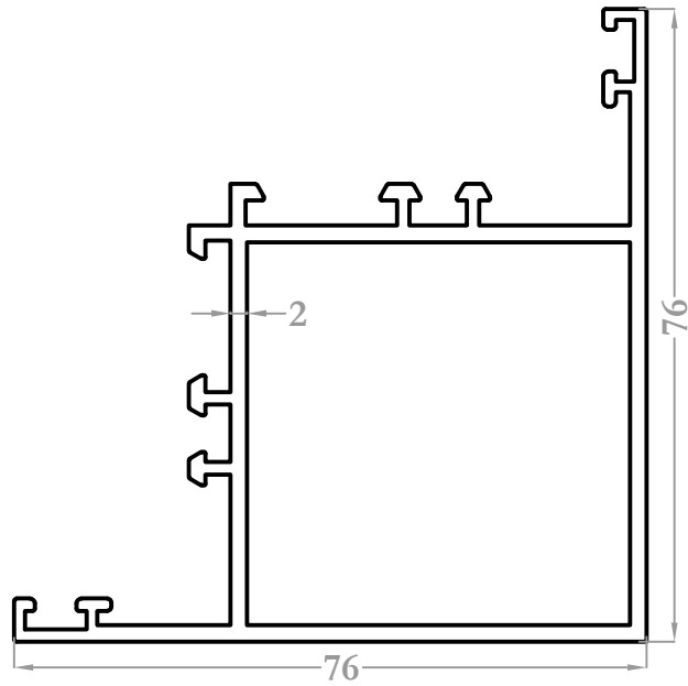
4539 1,582 kg/m
