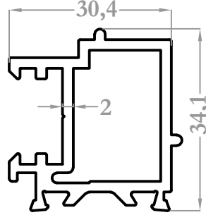
2623 0,776 kg/m
