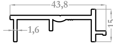
4535 0,380 kg/m
