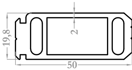
2599 0,597 kg/m
