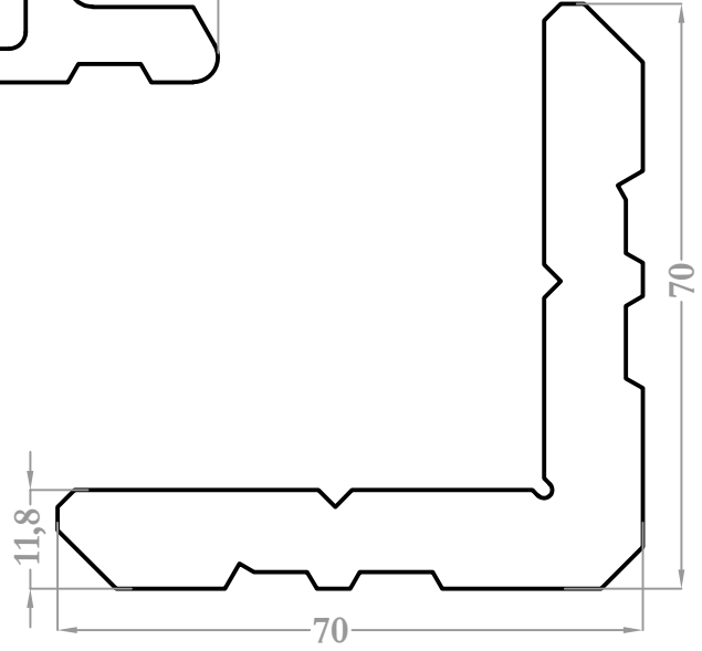
3036 3,672 kg/m
