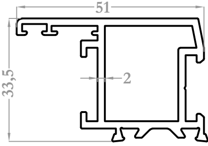
2604 0,921 kg/m
