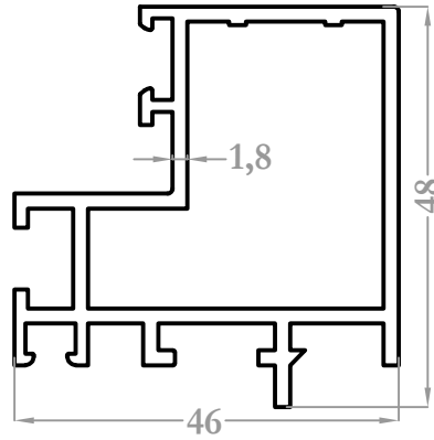
3501 1,020 kg/m
