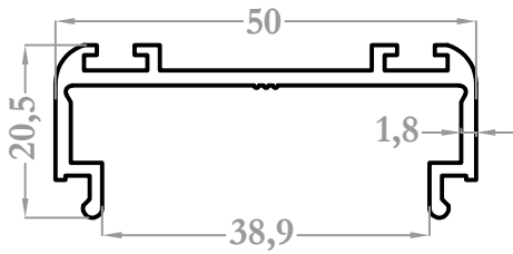
4666 0,501 kg/m
