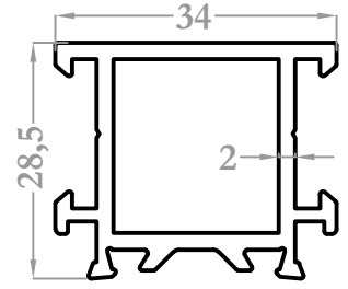
2590 0,702 kg/m
