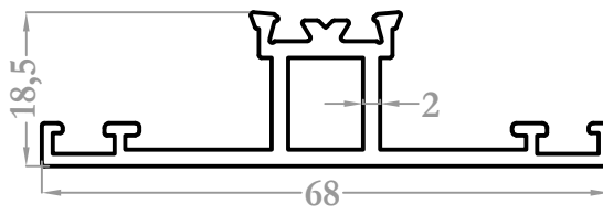
1945 0,697 kg/m
