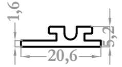
3504 0,152 kg/m
