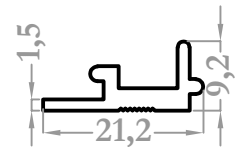
1721 0,196 kg/m
