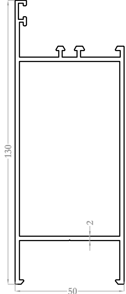
4533 1,910 kg/m
