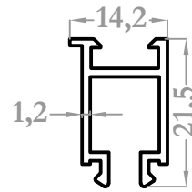
3027 0,210 kg/m
