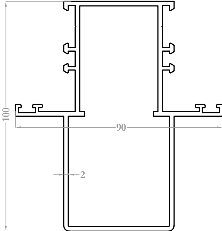
4532 2,054 kg/m
