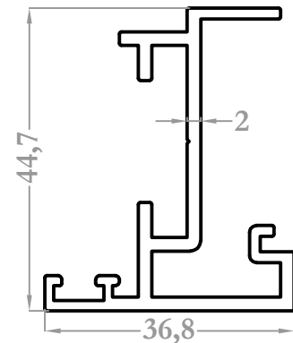
4536 0,735 kg/m
