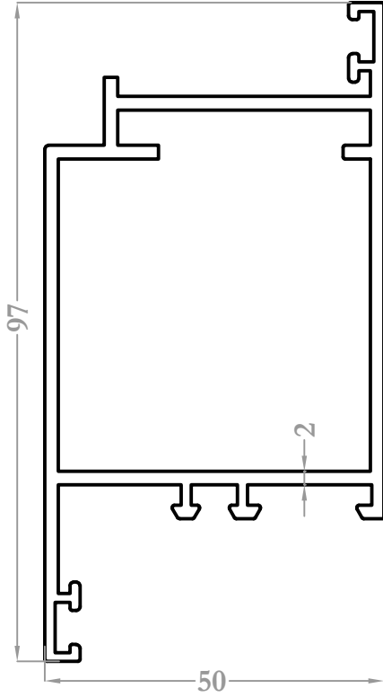
4534 1,558 kg/m
