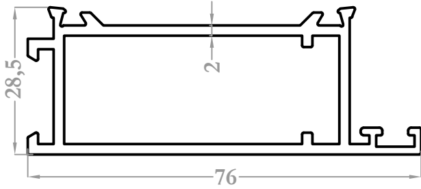
8718 1,120 kg/m
