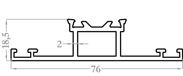
2602 0,791 kg/m
