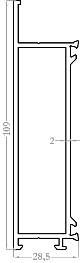
8700 1,401 kg/m
