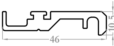
2599 0,597 kg/m
