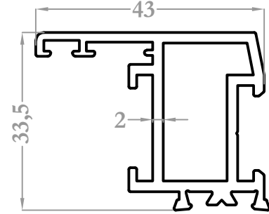
1946 0,818 kg/m
