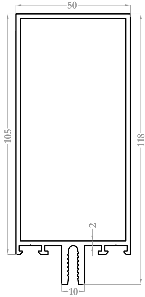
3211 1,950 kg/m
