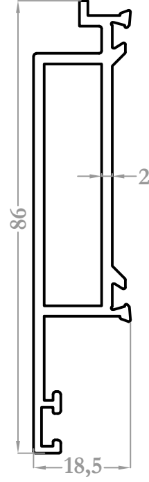
8717 0,978 kg/m
