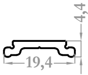
3028 0,128 kg/m
