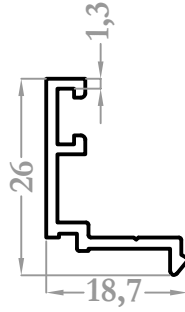
3013 0,211 kg/m
