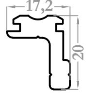
3505 0,370 kg/m
