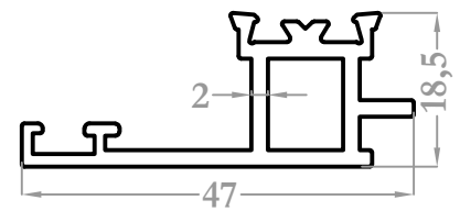
1943 0,563 kg/m
