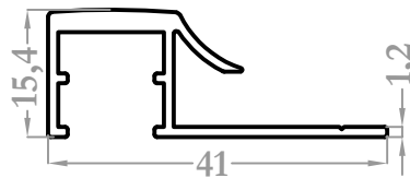
8369 0,321 kg/m
