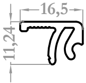
8507 0,181 kg/m
