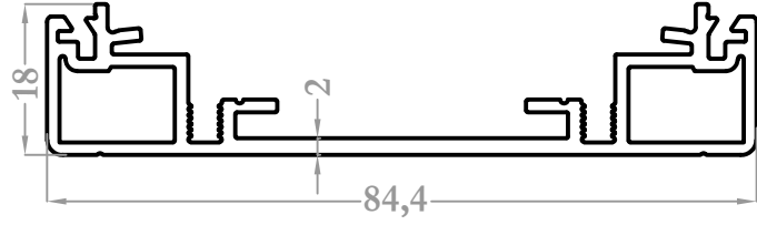
8505 0,926 kg/m
