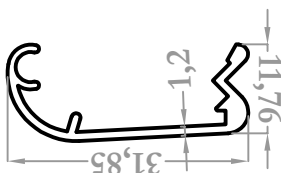
8321 0,210 kg/m
