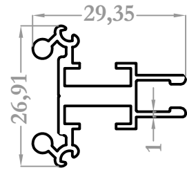
8308 0,448 kg/m
