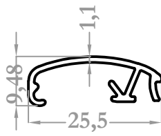
8433 0,153 kg/m
