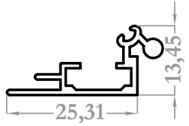
8198 0,210 kg/m
