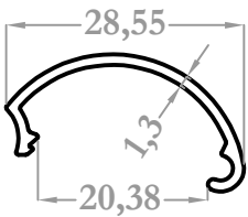
8326 0,171 kg/m
