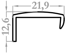
8090 0,171 kg/m
