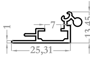
8198 0,210 kg/m
