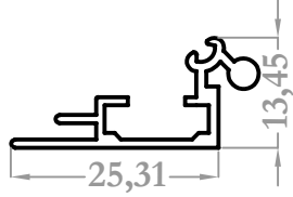
8198 0,210 kg/m
