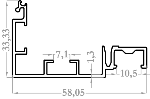
8502 0,550 kg/m
