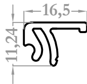
8508 0,182 kg/m
