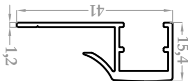
8369 0,321 kg/m
