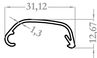
8397 0,165 kg/m
