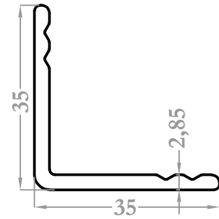
8817 0,492 kg/m
