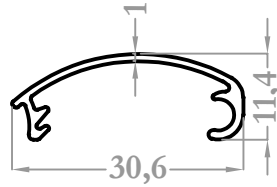
8428 0,151 kg/m
