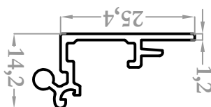
8100 0,221 kg/m
