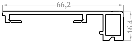
8784 0,627 kg/m
