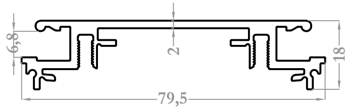
8506 0,902 kg/m
