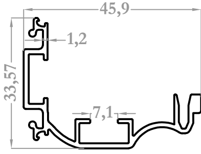
8501 0,447 kg/m
