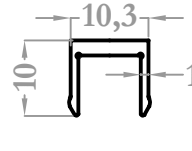
37044 0,088 kg/m
