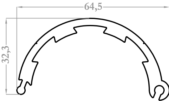
37033 1,086 kg/m
