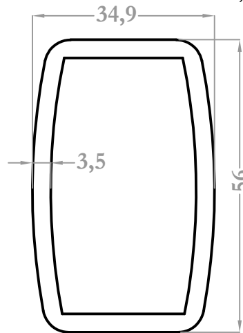
37034 1,461 kg/m
