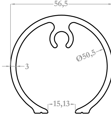
37027 1,533 kg/m
