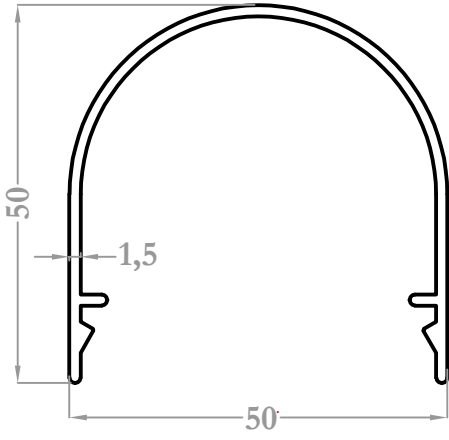
1803 0,556 kg/m
