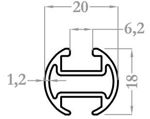
9400 0,280 kg/m
