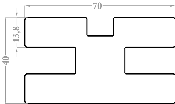
37051 5,741 kg/m
