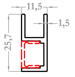
37045 0,231 kg/m
