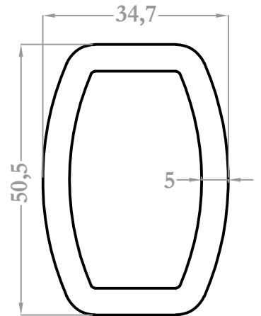
37035 1,782 kg/m
