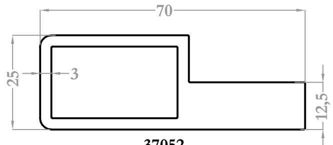
37052 1,978 kg/m
