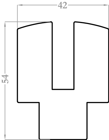
1810 4,129 kg/m
