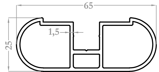
37042 0,853 kg/m
