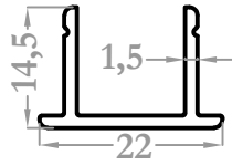
8762 0,190 kg/m
