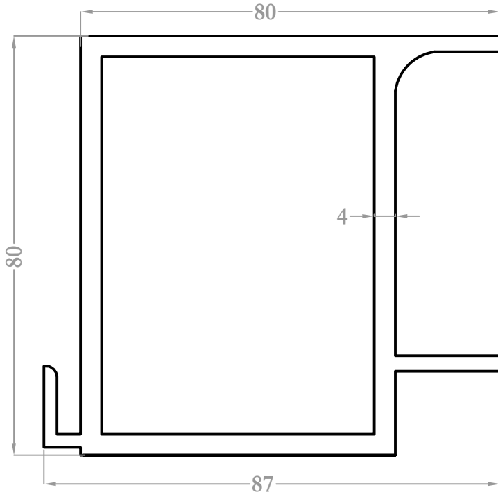
9384 3,360 kg/m
