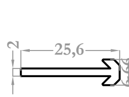
9531 0,178 kg/m
