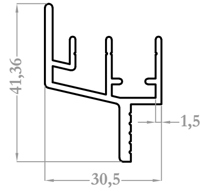
37127 0,569 kg/m
