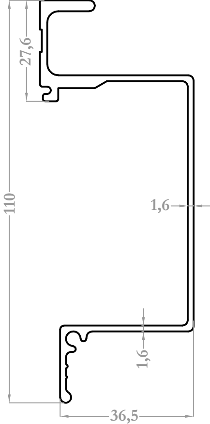
9188 1,086 kg/m
