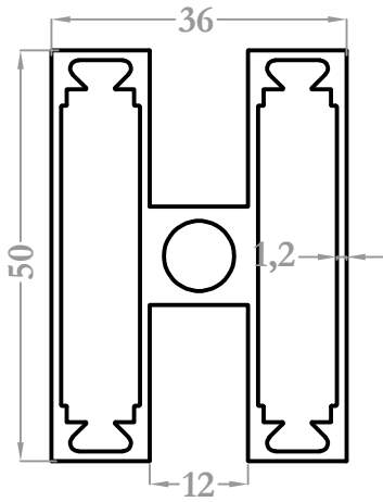
9342 1,176 kg/m
