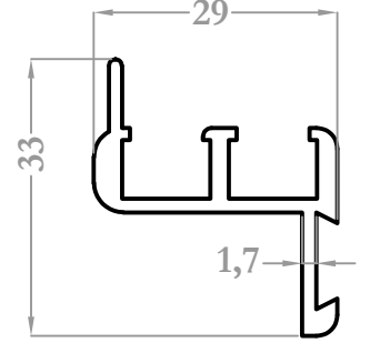
37131 0,438 kg/m
