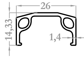
9619 0,238 kg/m
