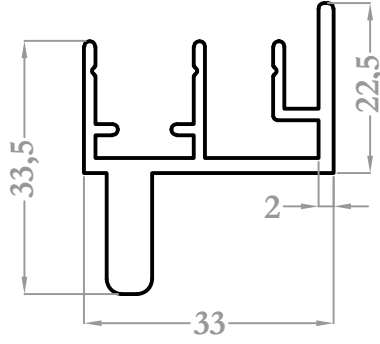
37120 0,750 kg/m
