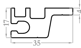
9468 0,778 kg/m
