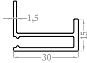
9227 0,379 kg/m
