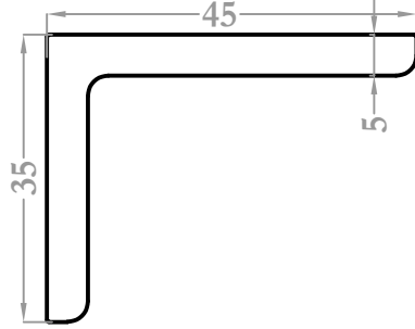
9570 1,012 kg/m
