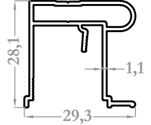
8657 0,365 kg/m
