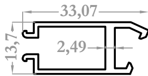
9108 0,320 kg/m
