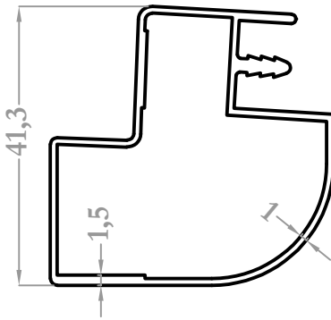
9218 0,527 kg/m
