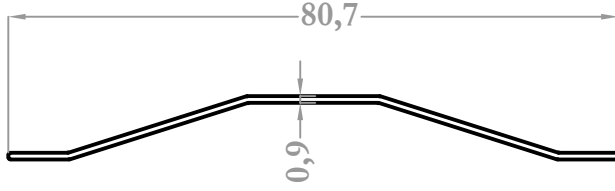
9115 0,202 kg/m
