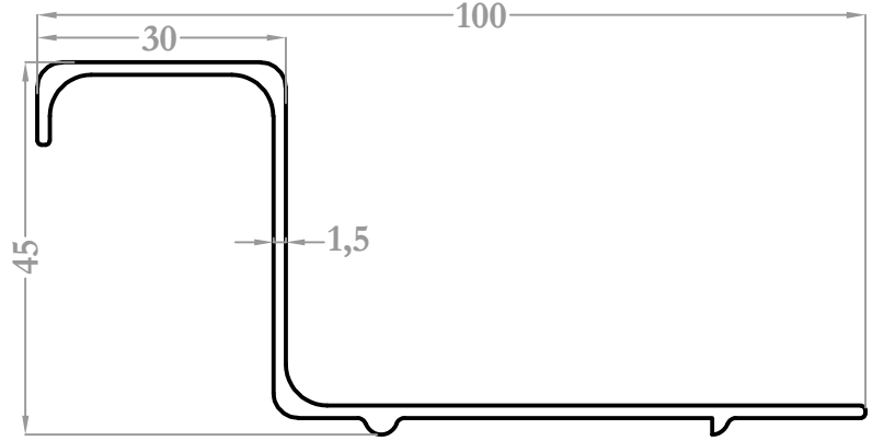
9273 0,664 kg/m
