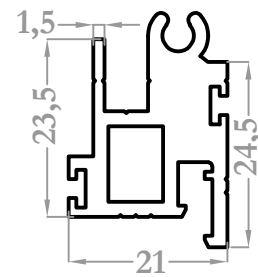
9644 0,749 kg/m
