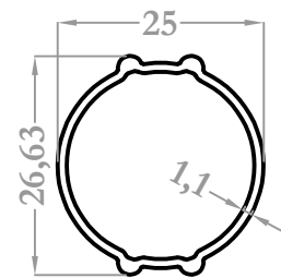
9467 0,251 kg/m
