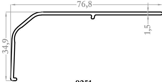
9251 0,425 kg/m
