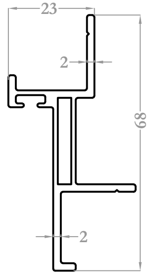
9276 0,681 kg/m
