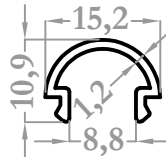
8673 0,105 kg/m
