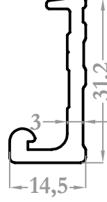
9133 0,396 kg/m
