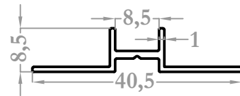
9393 0,161 kg/m
