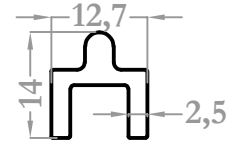
9337 0,212 kg/m
