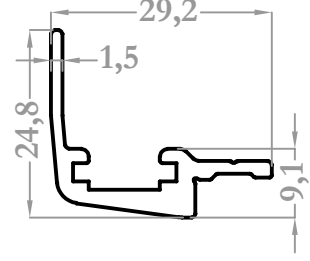
9134 0,349 kg/m
