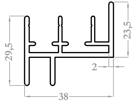
37121 0,707 kg/m
