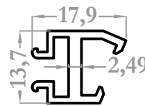
9109 0,219 kg/m
