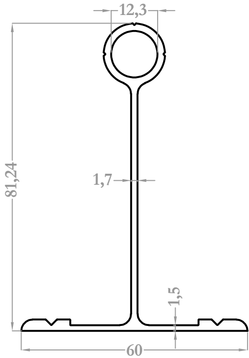
9386 0,878 kg/m
