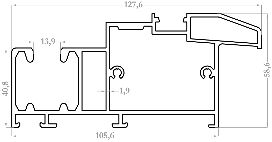
9207 2,750 kg/m
