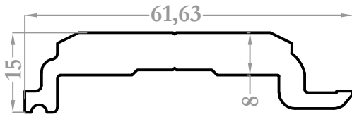
9466 1,157 kg/m
