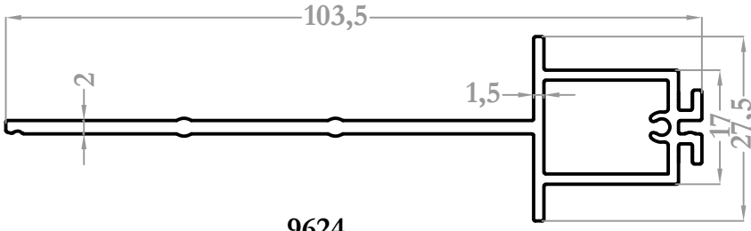
9624 0,827 kg/m
