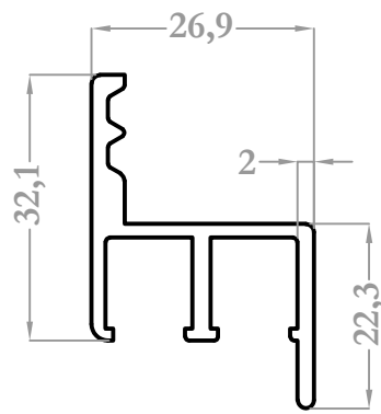
37126 0,526 kg/m
