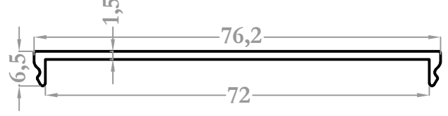
9325 0,348 kg/m
