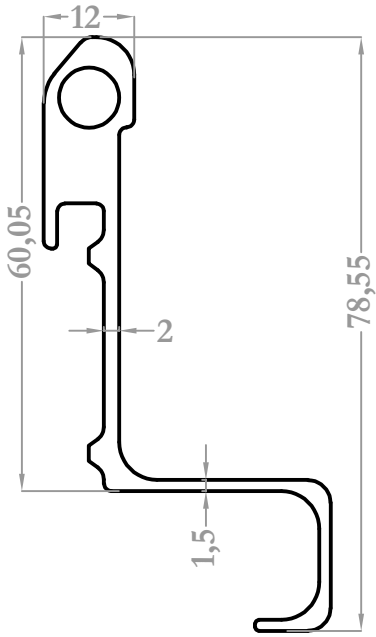
9270 0,990 kg/m
