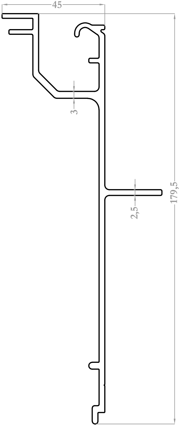
9090 2,098 kg/m
