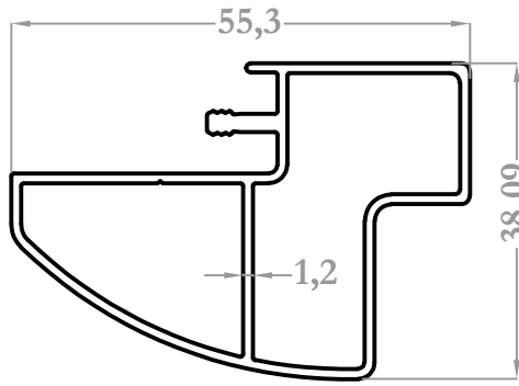
9219 0,677 kg/m
