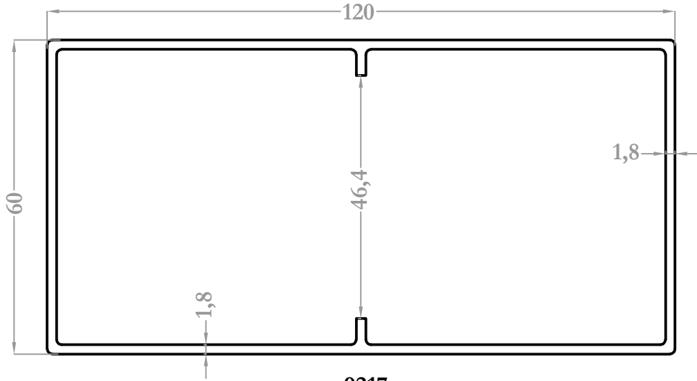
9217 1,772 kg/m
