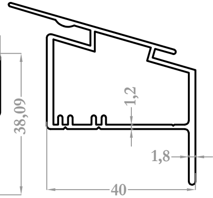
9220 0,676 kg/m
