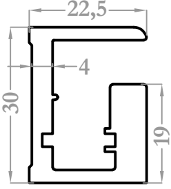
8640 0,826 kg/m
