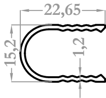
8672 0,170 kg/m
