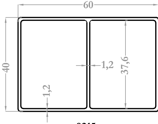
9215 0,758 kg/m
