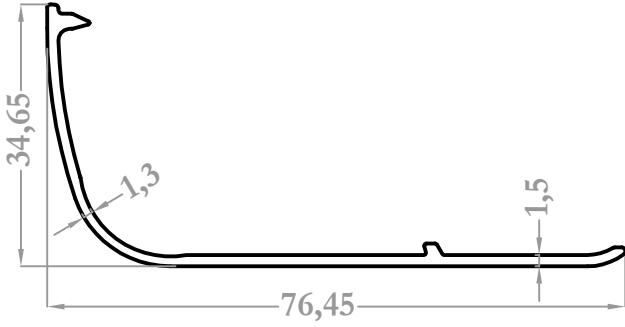
9198 0,430 kg/m
