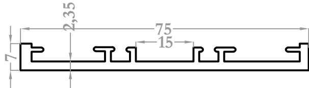
9070 0,650 kg/m
