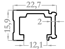
9355 0,356 kg/m
