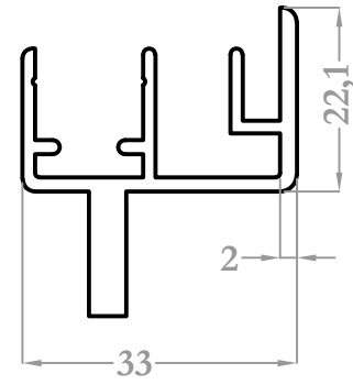
37124 0,649 kg/m
