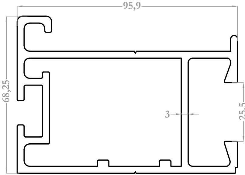
9450 3,266 kg/m
