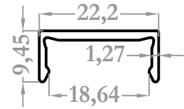
9354 0,152 kg/m
