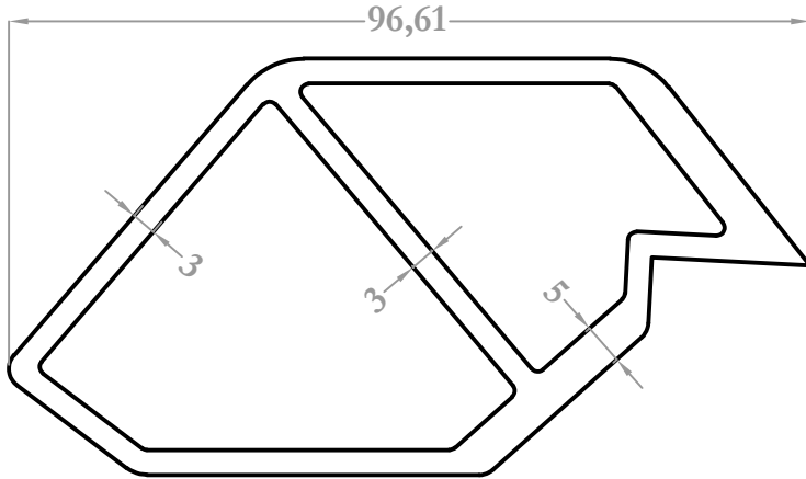
9104 2,514 kg/m
