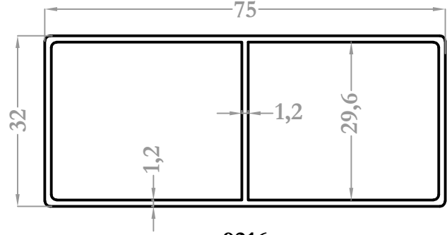
9216 0,777 kg/m
