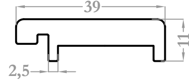
9167 0,765 kg/m
