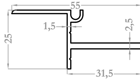
9261 0,425 kg/m
