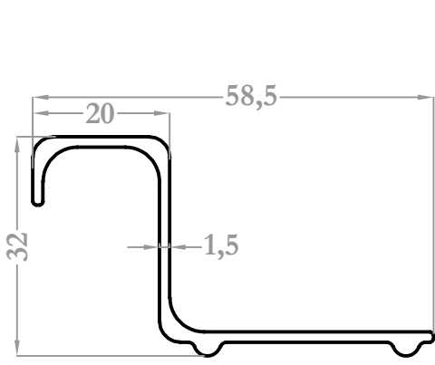
9272 0,451 kg/m
