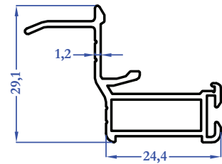
2208 0,381 kg/m
