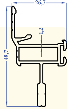
2205 0,487 kg/m
