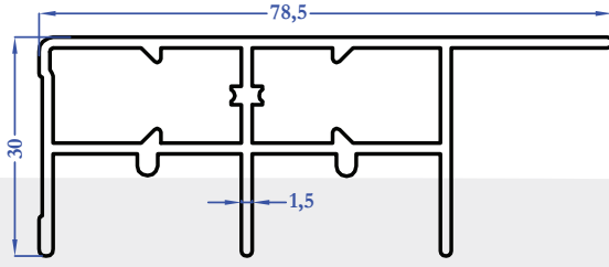
8546 0,972 kg/m
