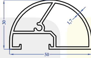
8782 0,756 kg/m
