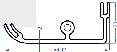
8778 0,515 kg/m
