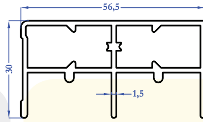
8547 0,880 kg/m
