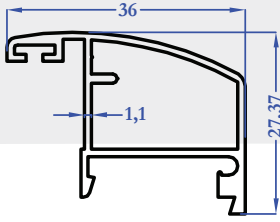
8862 0,392 kg/m
