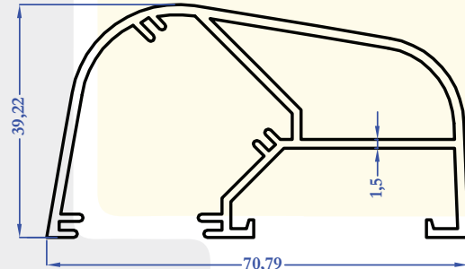
8609 1,003 kg/m
