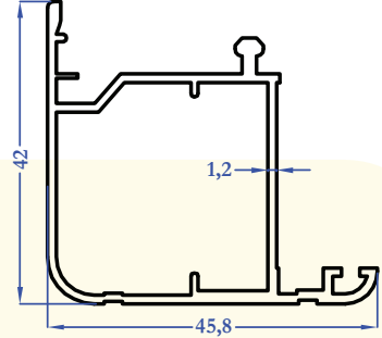
8783 0,595 kg/m
