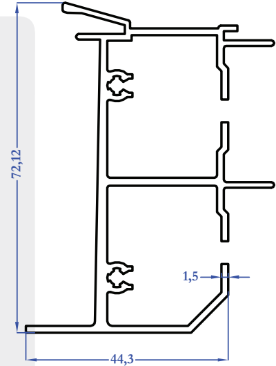
2202 1,232 kg/m
