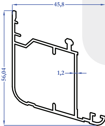
8642 0,620 kg/m
