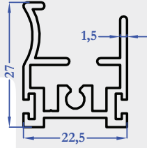
8863 0,475 kg/m
