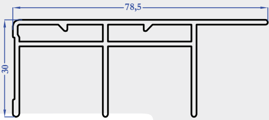
8548 0,897 kg/m
