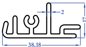
9264 0,499 kg/m
