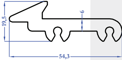
2209 1,118 kg/m
