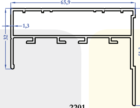
2201 1,232 kg/m
