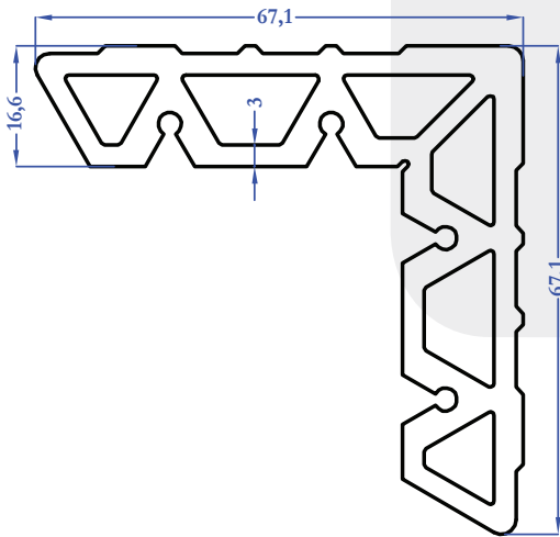
2206 2,833 kg/m
