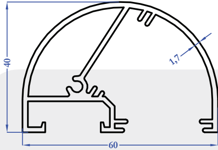
8781 0,937 kg/m
