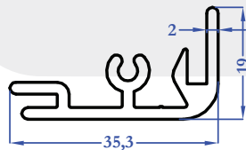
9265 0,476 kg/m
