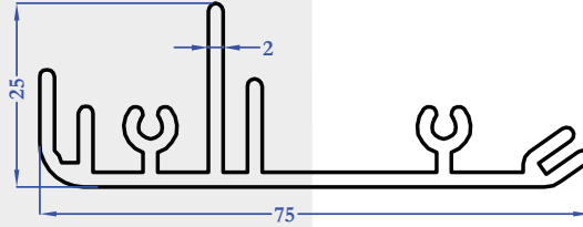
9263 0,940 kg/m
