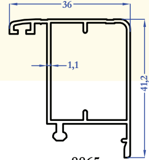
8865 0,488 kg/m
