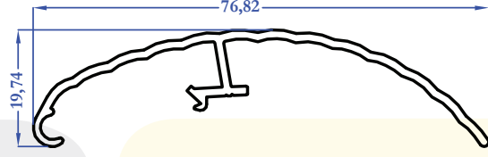
8488 0,458 kg/m
