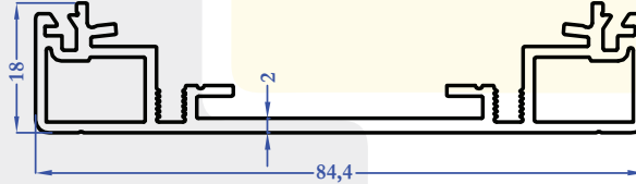
8505 0,926 kg/m
