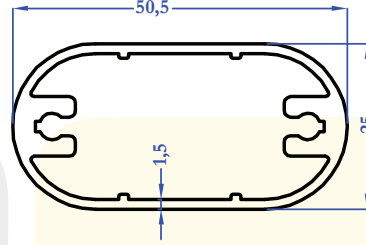
R9028 0,792 kg/m
