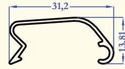
8088 0,164 kg/m
