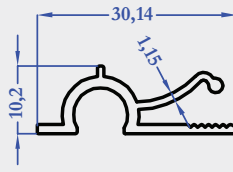
E1020 0,224 kg/m
