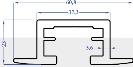
R9318 0,418 kg/m
