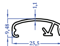
8433 0,153 kg/m
