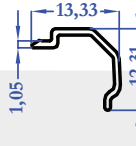
8087 0,062 kg/m
