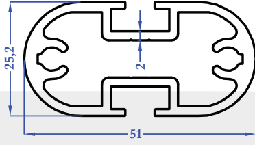
8485 1,084 kg/m
