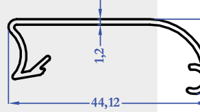
8242 0,266 kg/m
