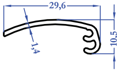
E1021 0,161 kg/m
