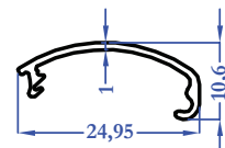
8243 0,107 kg/m
