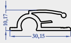
8076 0,267 kg/m
