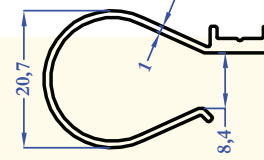
8504 0,234 kg/m
