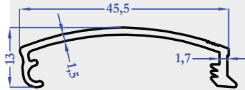
8360 0,286 kg/m
