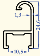
8201 0,216 kg/m
