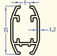
8203 0,267 kg/m
