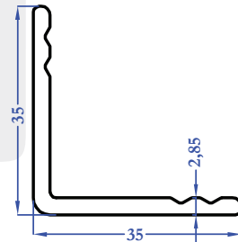
8817 0,492 kg/m
