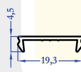
8084 0,074 kg/m
