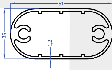
8371 0,664 kg/m
