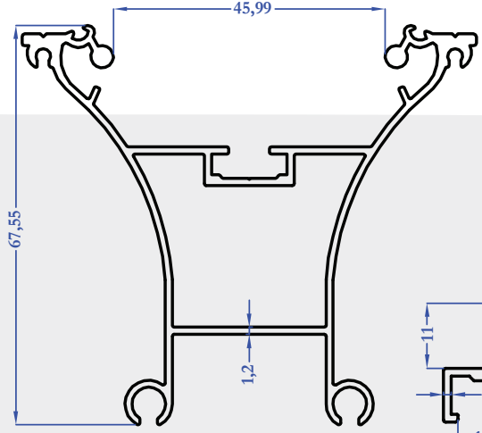
8119 1,072 kg/m
