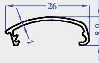
E2298 0,106 kg/m
