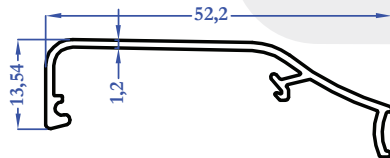
8500 0,275 kg/m
