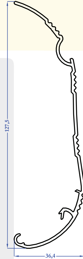
8489 0,818 kg/m
