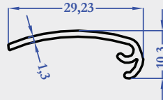
E2297 0,146 kg/m
