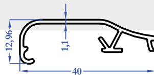
8432 0,215 kg/m
