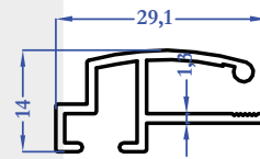
E2296 0,260 kg/m
