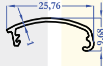
E1615 0,108 kg/m
