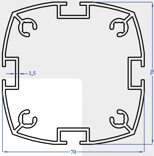
8486 1,704 kg/m
