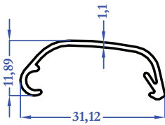
8397 0,165 kg/m
