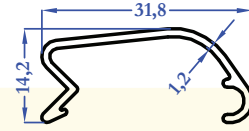
8098 0,190 kg/m
