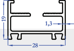
8031 0,336 kg/m
