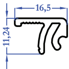
8507 0,181 kg/m
