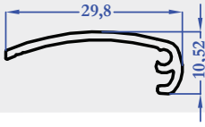
8075 0,157 kg/m
