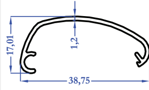
8430 0,210 kg/m
