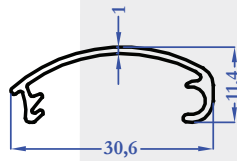
8428 0,151 kg/m
