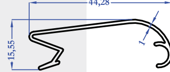
E1601 0,224 kg/m
