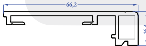
8784 0,627 kg/m
