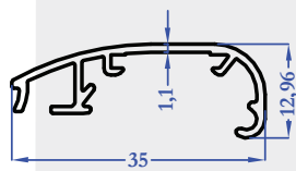
8435 0,215 kg/m
