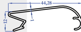
8361 0,224 kg/m
