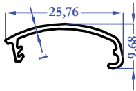
8322 0,108 kg/m
