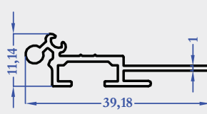
8429 0,234 kg/m
