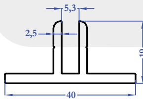
R9333 0,536 kg/m
