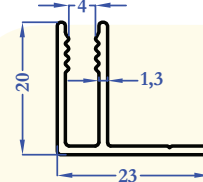
M5048 0,220 kg/m
