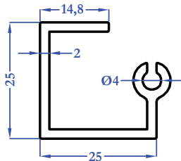
M5025 0,456 kg/m
