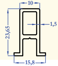
R9172 0,282 kg/m
