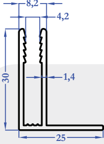
R9238 0,330 kg/m
