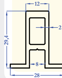
R9097 0,543 kg/m
