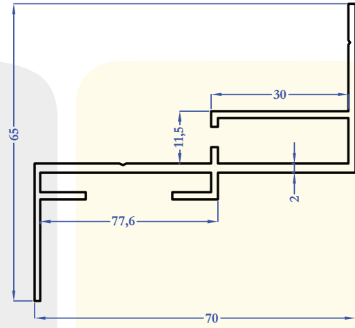
R9121 0,855 kg/m
