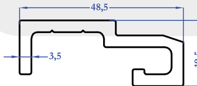
M5286 0,847 kg/m
