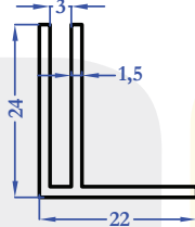
M5419 0,273 kg/m
