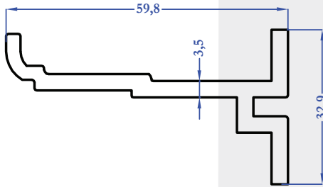
M5094 0,976 kg/m
