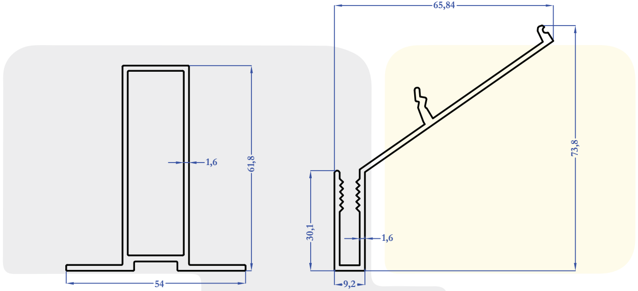
R9209 0,886 kg/m
