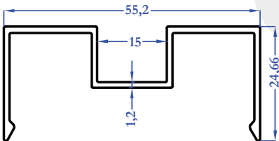
R9119 0,440 kg/m
