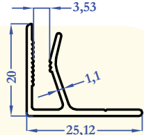
E1743 0,214 kg/m
