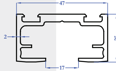
M5782 0,879 kg/m
