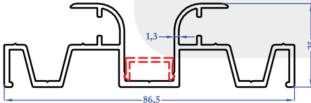
M5405 0,886 kg/m
