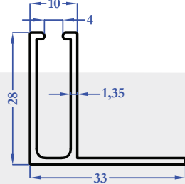
R9267 0,332 kg/m
