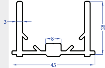
M5026 0,828 kg/m
