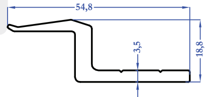
M5287 0,637 kg/m
