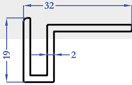
R9084 0,346 kg/m
