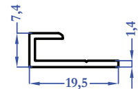
E2989 0,113 kg/m
