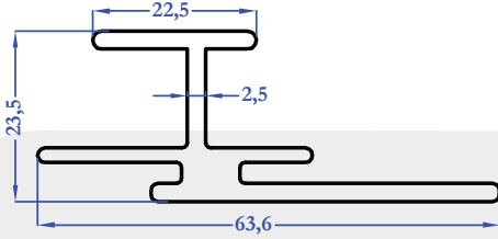
R9118 0,832 kg/m
