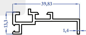
R9210 0,324 kg/m
