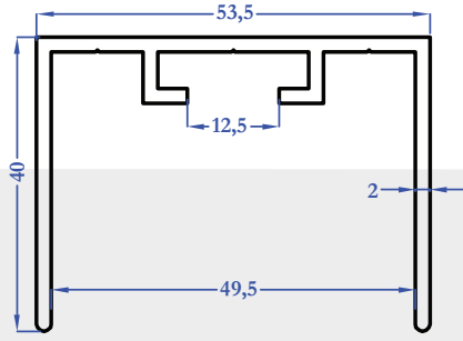
9122 0,283 kg/m
