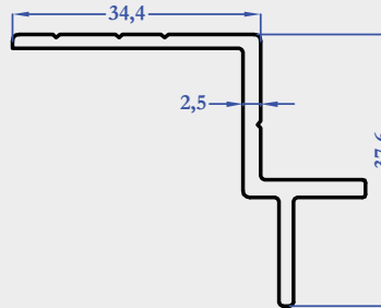
9022 0,501 kg/m
