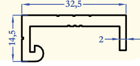
9160 0,460 kg/m
