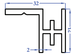
8073 0,504 kg/m
