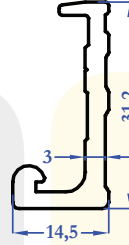
9133 0,396 kg/m
