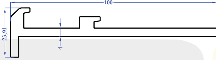
9166 1,478 kg/m
