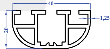
8711 0,665 kg/m
