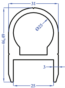
9562 1,208 kg/m
