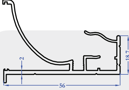
9221 0,681 kg/m
