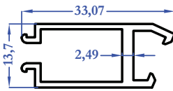
9108 0,320 kg/m
