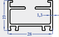
8750 0,325 kg/m
