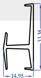
8802 0,260 kg/m
