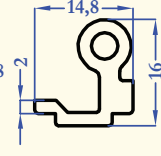
8444 0,246 kg/m
