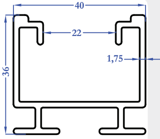
8635 0,771 kg/m
