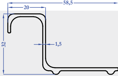
9272 0,451 kg/m
