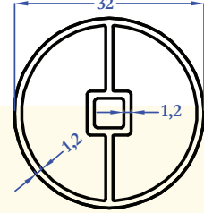
8678 0,466 kg/m
