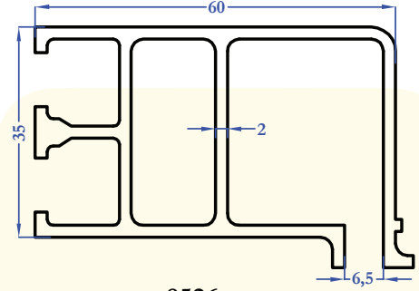
8526 1,365 kg/m
