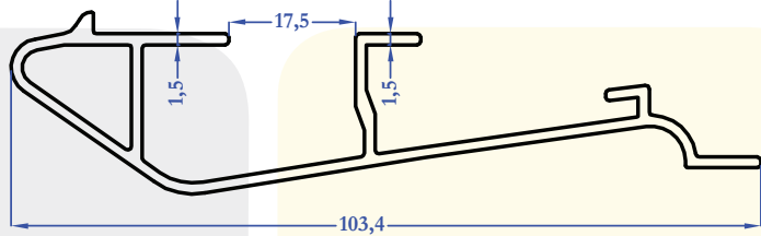
9223 0,807 kg/m
