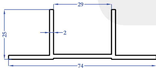
8060 0,650 kg/m
