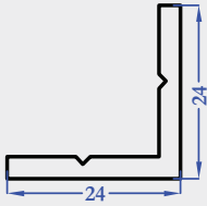
8440 0,360 kg/m
