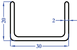
8083 0,355 kg/m
