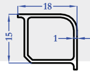
9579 0,163 kg/m
