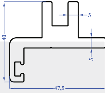
8953 1,505 kg/m
