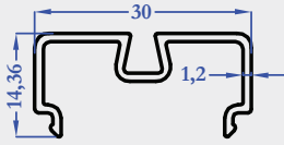
8392 0,275 kg/m
