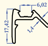
8543 0,183 kg/m
