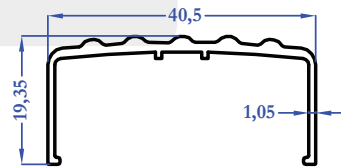
8078 0,289 kg/m
