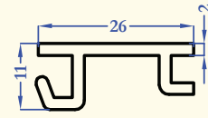
8899 0,287 kg/m
