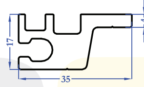
9468 0,778 kg/m
