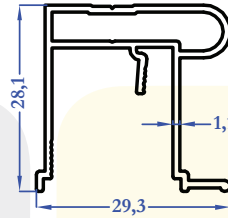
8657 0,365 kg/m
