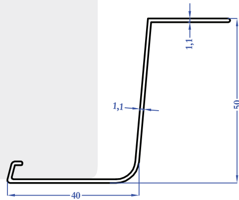
9238 0,352 kg/m
