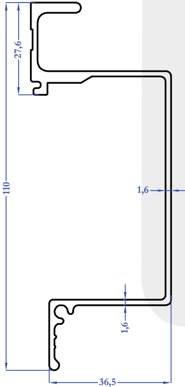
9188 1,086 kg/m
