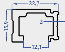
9355 0,356 kg/m
