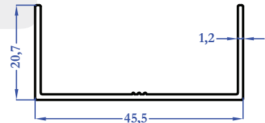
9015 0,273 kg/m
