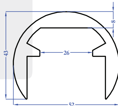
9568 1,708 kg/m
