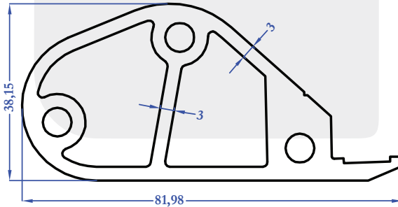
8921 2,413 kg/m
