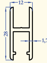
9571 0,306 kg/m
