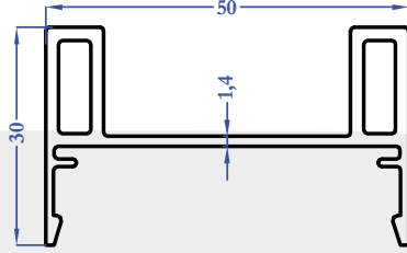
8641 0,650 kg/m
