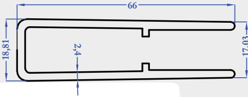
8668 0,280 kg/m
