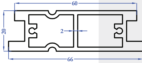
8003 1,263 kg/m
