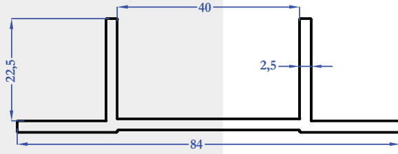
8059 0,874 kg/m
