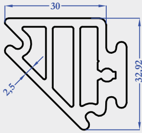
8531 1,179 kg/m
