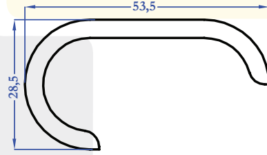
8436 0,907 kg/m
