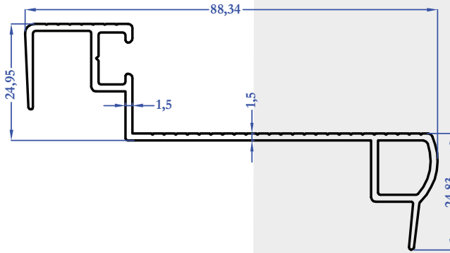
8897 0,731 kg/m
