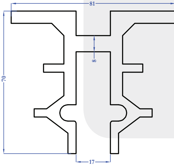
8364 0,999 kg/m
