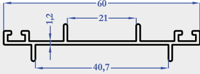
M5346 0,315 kg/m
