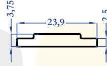
8633 0,208 kg/m
