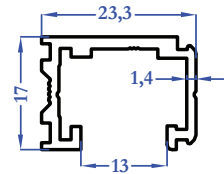
8596 0,294 kg/m
