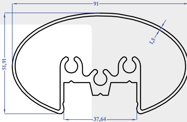
8401 1,787 kg/m
