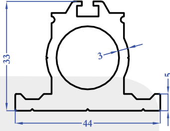
8427 1,333 kg/m
