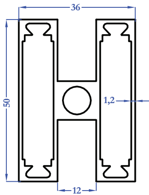
9342 1,176 kg/m
