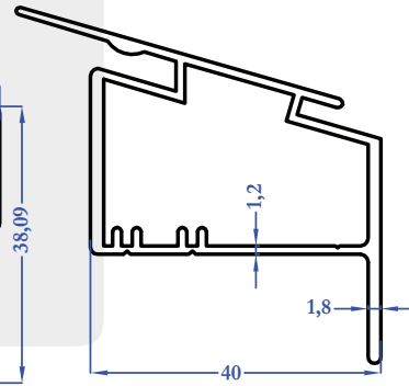
9220 0,676 kg/m
