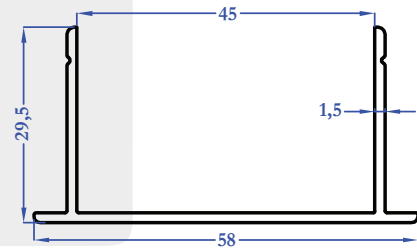
8761 0,458 kg/m
