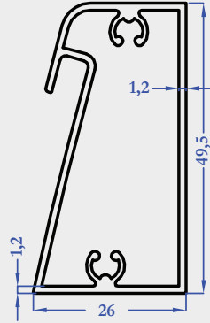
8732 0,582 kg/m
