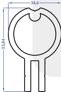
8337 1,424 kg/m
