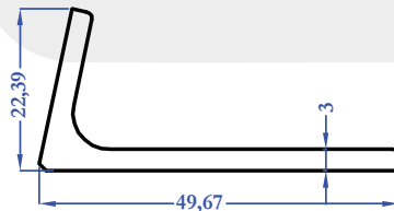
9014 0,580 kg/m
