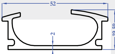
8351 0,633 kg/m
