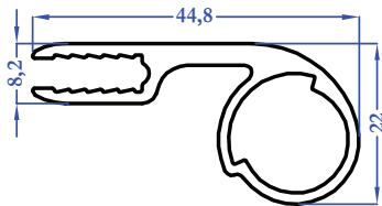
9224 0,580 kg/m
