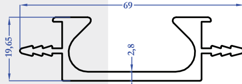
8841 0,907 kg/m
