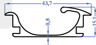
9662 0,369 kg/m
