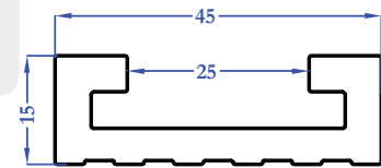
E2337 0,988 kg/m
