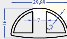
9285 0,556 kg/m
