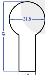
9463 1,596 kg/m
