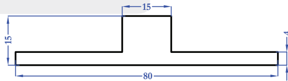
8623 1,314 kg/m
