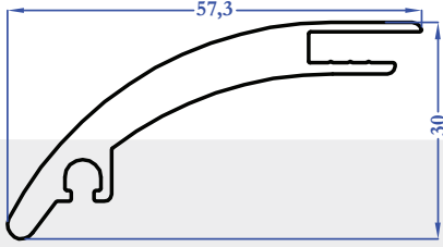
11315 0,915 kg/m
