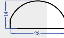
E1520 0,863 kg/m
