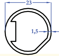
9136 0,365 kg/m
