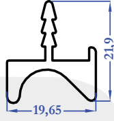
8842 0,360 kg/m
