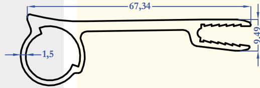
9283 0,794 kg/m
