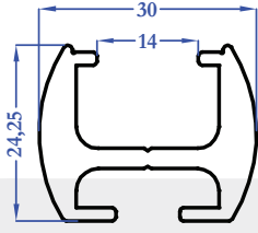
M5393 0,775 kg/m
