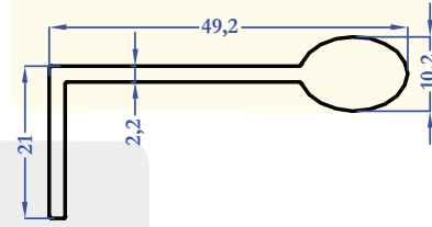
8653 0,637 kg/m
