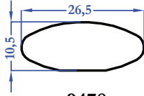
9478 0,601 kg/m
