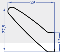
8631 0,802 kg/m
