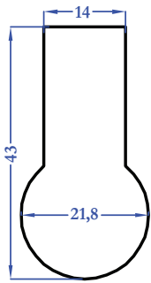
9448 1,846 kg/m
