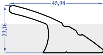
8616 0,967 kg/m
