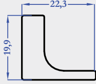
E1304 0,513 kg/m
