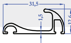
9845 0,236 kg/m
