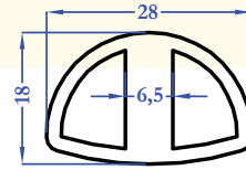
9286 0,617 kg/m
