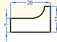
9139 0,449 kg/m
