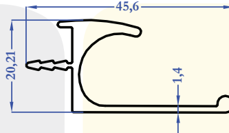
9424 0,438 kg/m
