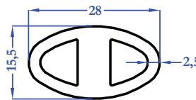
9427 0,614 kg/m
