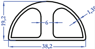
11538 0,662 kg/m
