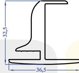
11317 0,915 kg/m
