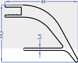
11314 0,867 kg/m
