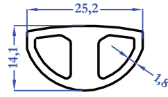
11266 0,472 kg/m
