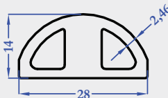
9375 0,604 kg/m
