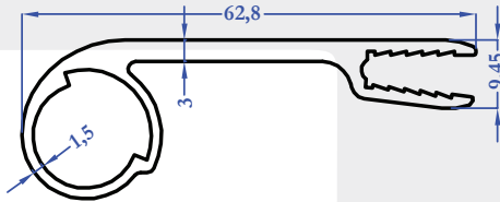
9284 0,743 kg/m
