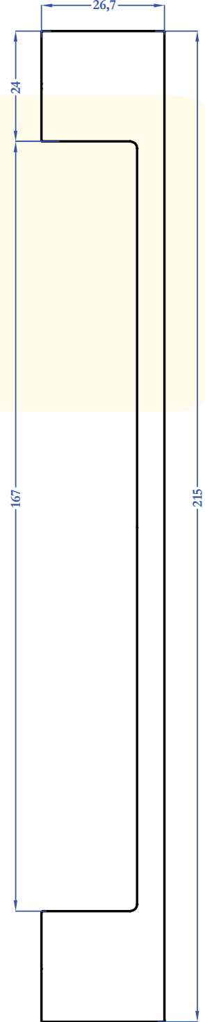
10218 6,146 kg/m
