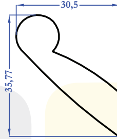
8629 1,607 kg/m
