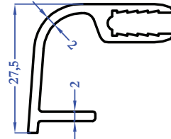
9307 0,434 kg/m
