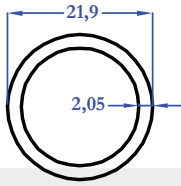
508 0,346 kg/m
