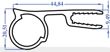
8962 0,557 kg/m
