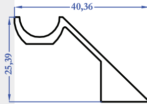
8276 0,471 kg/m
