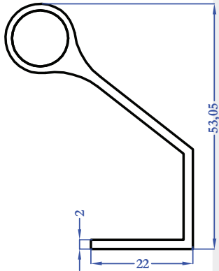
8274 0,613 kg/m
