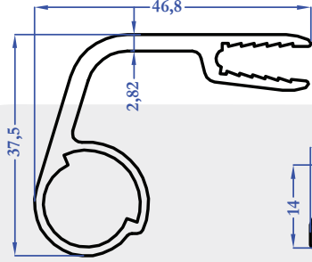
9310 0,731 kg/m
