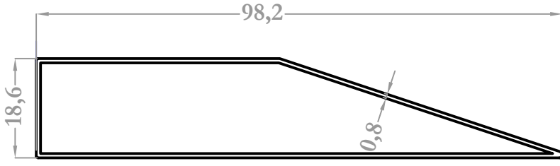
37132 0,470 kg/m
