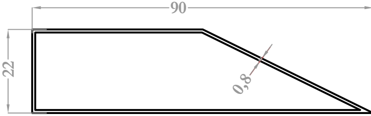
9171 0,493 kg/m
