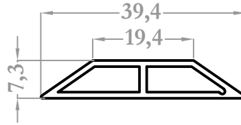
37133 0,268 kg/m
