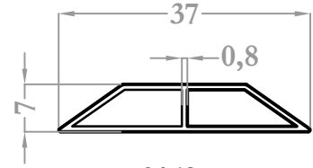
9152 0,174 kg/m
