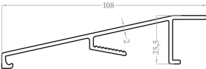
37083 0,932 kg/m
