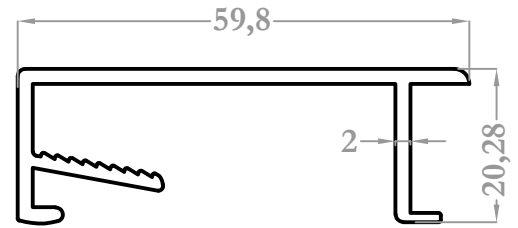
37084 0,649 kg/m
