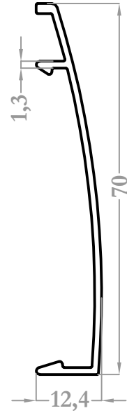
37082 0,335 kg/m
