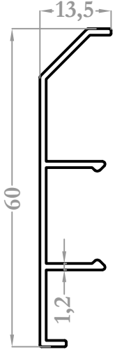
37079 0,497 kg/m
