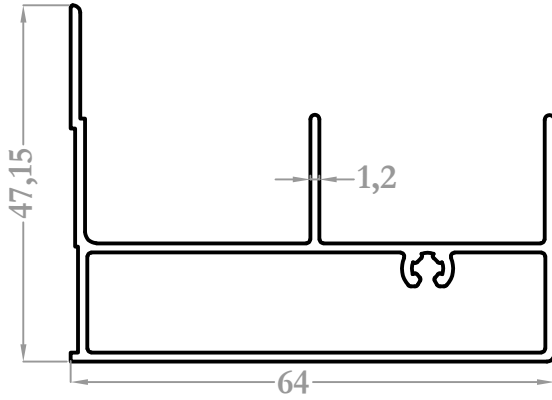
2204 0,771 kg/m
