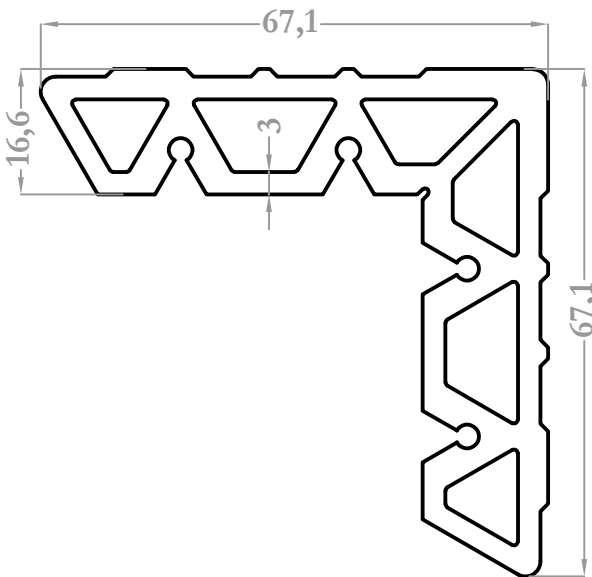
2206 2,833 kg/m
