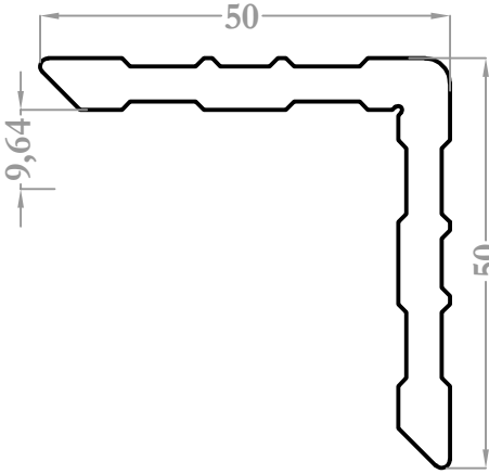
2200 1,293 kg/m
