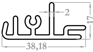
9264 0,499 kg/m
