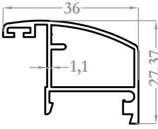
8862 0,392 kg/m
