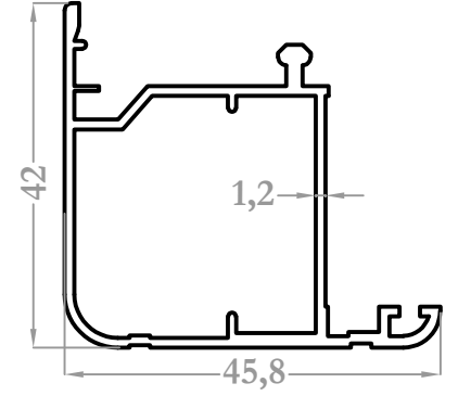
8783 0,595 kg/m
