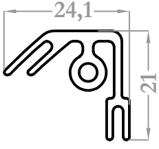
8779 0,345 kg/m
