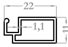
1909 0,194 kg/m
