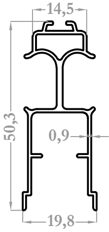
37092 0,380 kg/m
