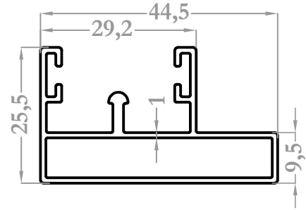
37097 0,485 kg/m
