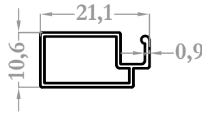
37091 0,139 kg/m
