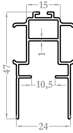
37093 0,436 kg/m
