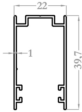
8706 0,323 kg/m
