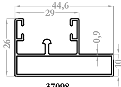
37098 0,426 kg/m
