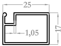
1910 0,246 kg/m
