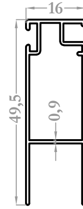
37094 0,348 kg/m
