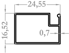
37089 0,164 kg/m
