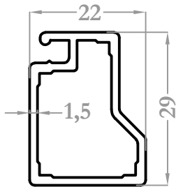
1911 0,424 kg/m
