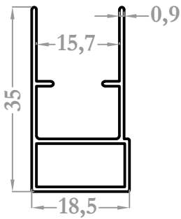
37095 0,267 kg/m
