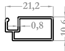
1922 0,139 kg/m
