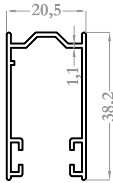
37086 0,336 kg/m
