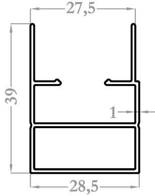
37096 0,396 kg/m
