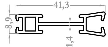
8705 0,342 kg/m
