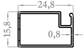
37090 0,184 kg/m
