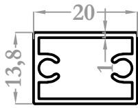
37087 0,223 kg/m
