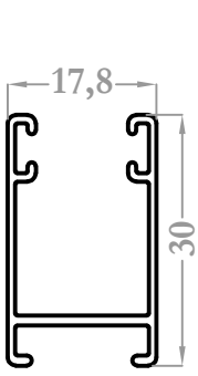
37085 0,247 kg/m
