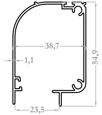
8708 0,562 kg/m
