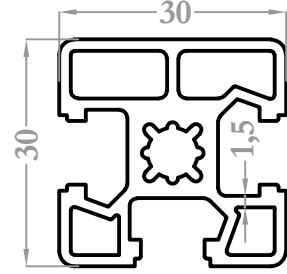
9052 0,906 kg/m
