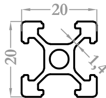
9053 0,421 kg/m
