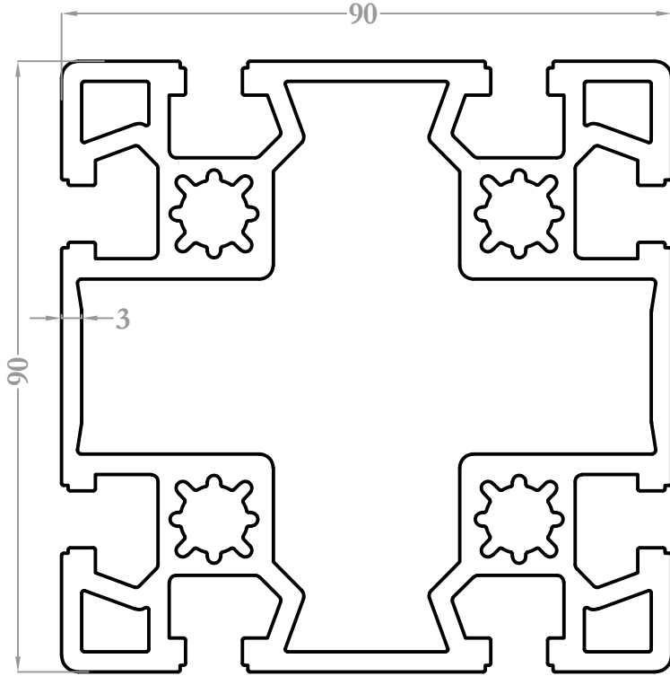
9059 6,138 kg/m
