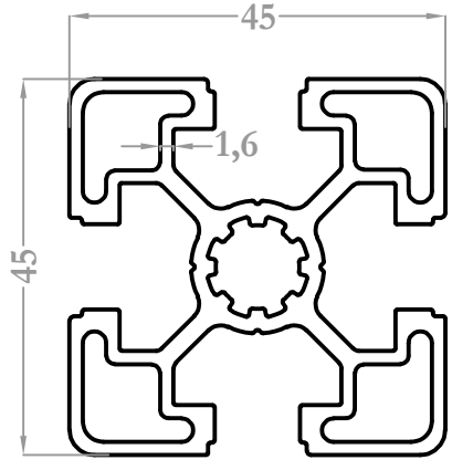
9348 1,598 kg/m
