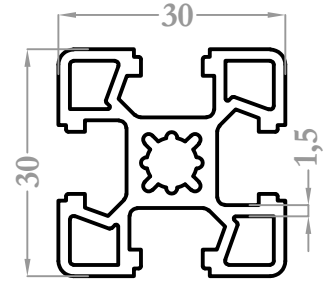
9057 0,878 kg/m
