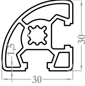
9050 0,794 kg/m
