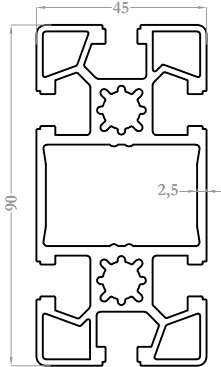
9055 3,158 kg/m
