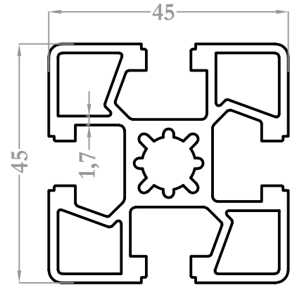
9058 1,766 kg/m
