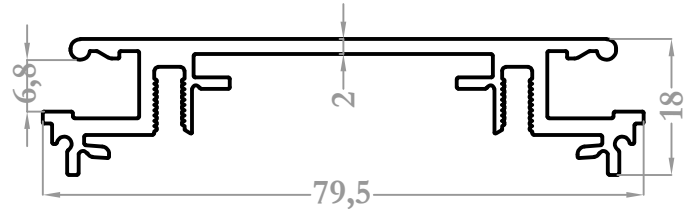
8506 0,902 kg/m
