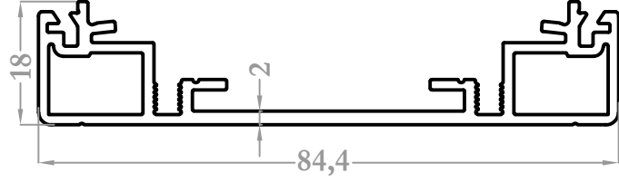
8505 0,926 kg/m
