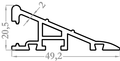
8032 0,577 kg/m
