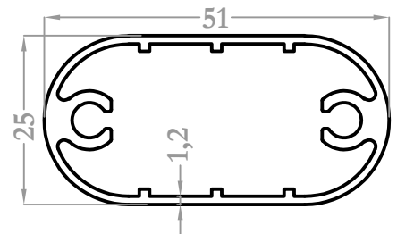
8371 0,664 kg/m
