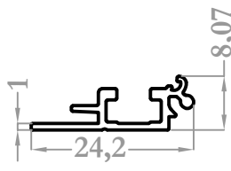
8097 0,138 kg/m
