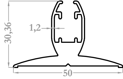
8849 0,712 kg/m
