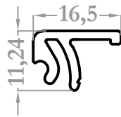
8508 0,182 kg/m
