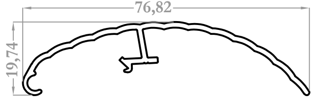
8488 0,458 kg/m
