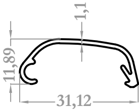
8397 0,165 kg/m
