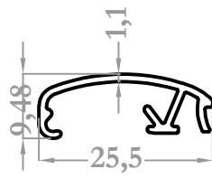
8433 0,153 kg/m
