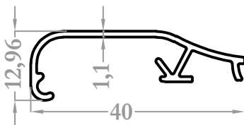
8432 0,215 kg/m
