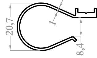
8504 0,234 kg/m
