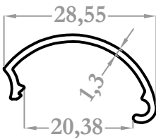
8326 0,171 kg/m
