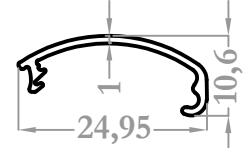
8243 0,107 kg/m
