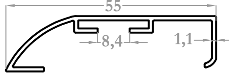
8204 0,294 kg/m
