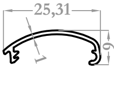
8099 0,104 kg/m
