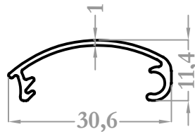
8428 0,151 kg/m
