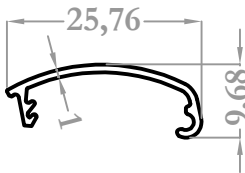
8322 0,108 kg/m
