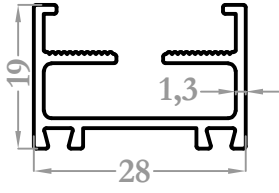
8031 0,336 kg/m
