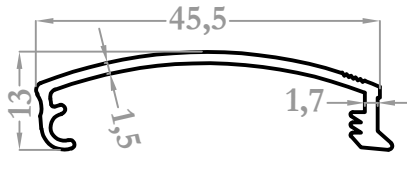
8360 0,286 kg/m
