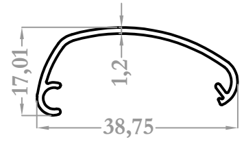
8430 0,210 kg/m
