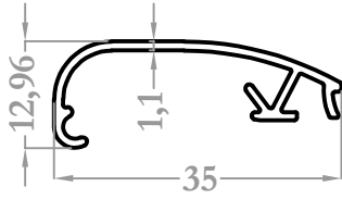
8434 0,197 kg/m
