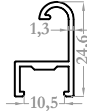
8201 0,216 kg/m
