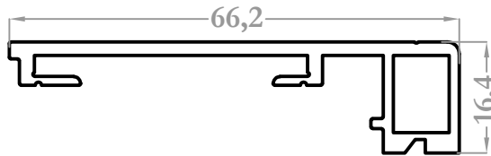
8784 0,627 kg/m
