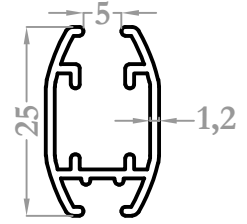
8203 0,267 kg/m
