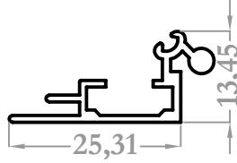
8198 0,210 kg/m
