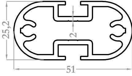
8485 1,084 kg/m
