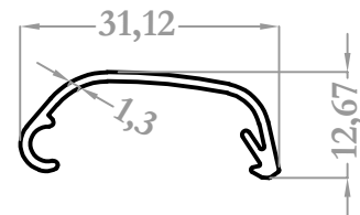
8397 0,165 kg/m
