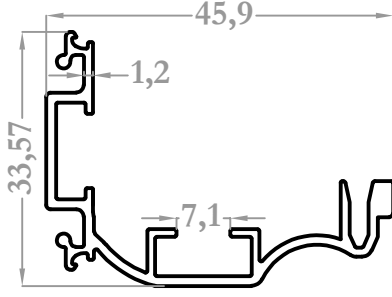
8501 0,447 kg/m
