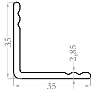
8817 0,492 kg/m
