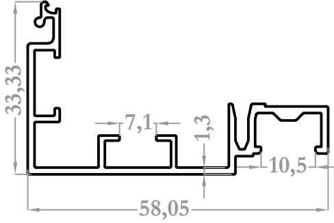
8502 0,550 kg/m
