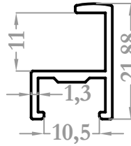
8200 0,200 kg/m
