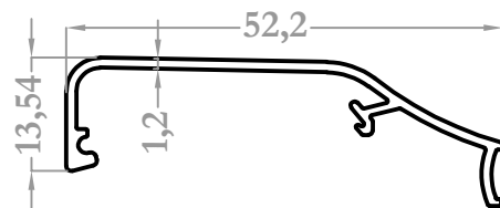
8500 0,275 kg/m
