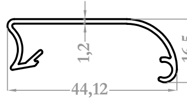
8242 0,266 kg/m
