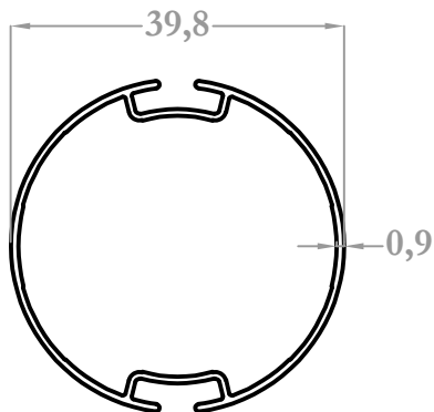
28041 0,332 kg/m
