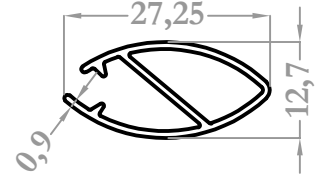
28012 0,182 kg/m
