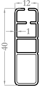
28027 0,331 kg/m
