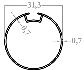
28043 0,210 kg/m
