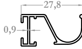
28016 0,185 kg/m
