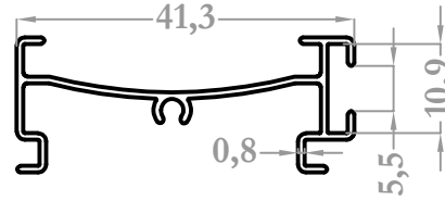
28047 0,223 kg/m
