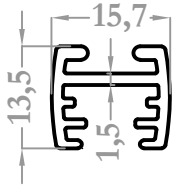
28011 0,226 kg/m
