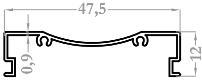
9376 0,225 kg/m
