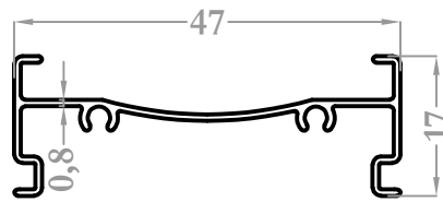
9379 0,240 kg/m
