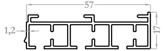
9397 0,604 kg/m
