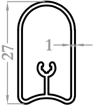
28013 0,230 kg/m
