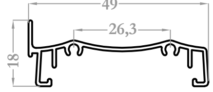
28046 0,290 kg/m
