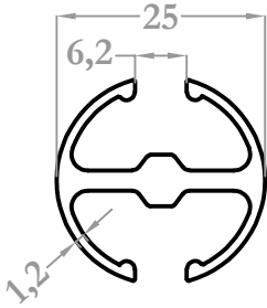
28018 0,429 kg/m
