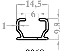
9068 0,105 kg/m
