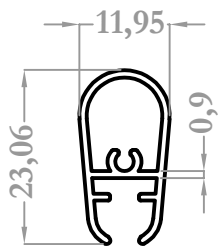
28061 0,193 kg/m
