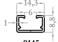
9145 0,102 kg/m
