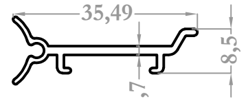
28056 0,216 kg/m
