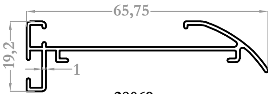
28069 0,358 kg/m
