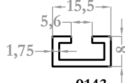
9143 0,163 kg/m
