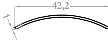
9460 0,117 kg/m
