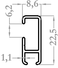
9067 0,153 kg/m
