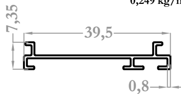
28062 0,148 kg/m
