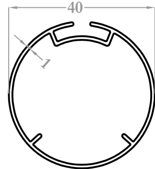
28040 0,398 kg/m
