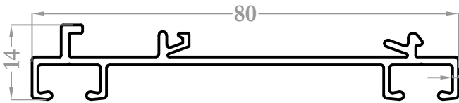
9613 0,548 kg/m
