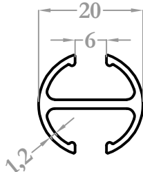
28019 0,249 kg/m
