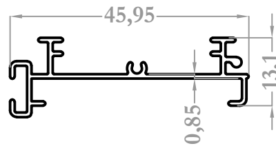
28050 0,223 kg/m
