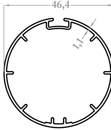
28038 0,521 kg/m
