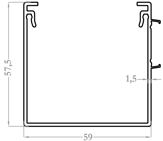
28071 0,819 kg/m
