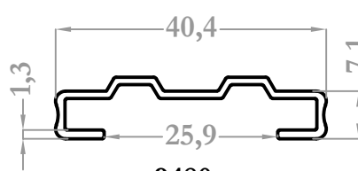
9480 0,211 kg/m
