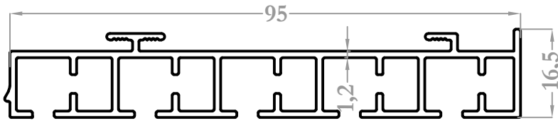
9399 0,935 kg/m
