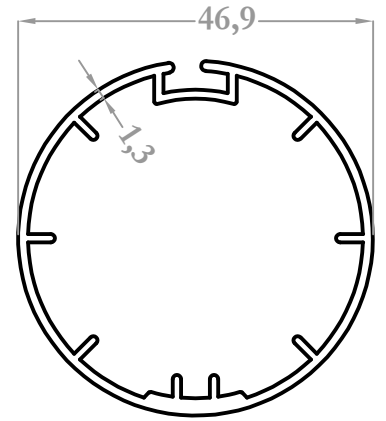
28039 0,658 kg/m
