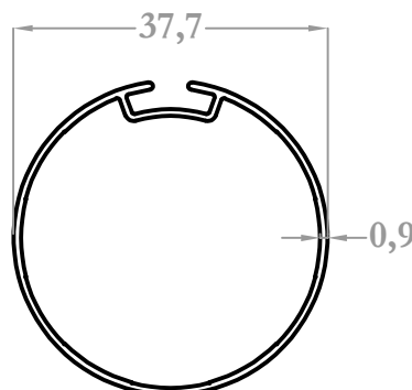
28042 0,291 kg/m
