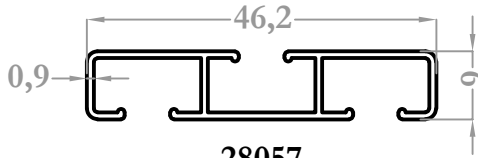
28057 0,254 kg/m
