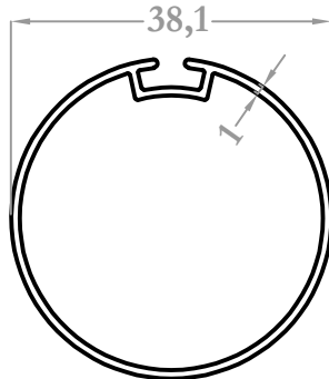
9202 0,344 kg/m
