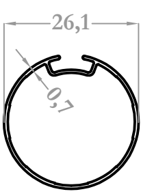
28044 0,151 kg/m
