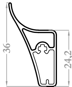
28029 0,104 kg/m
