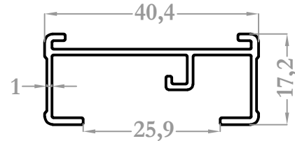
9481 0,309 kg/m
