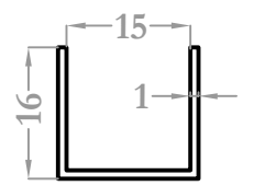
0005 0,128 kg/m
