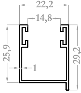
37020 0,648 kg/m
