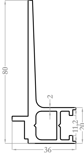
37017 1,308 kg/m
