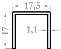
0001 0,146 kg/m
