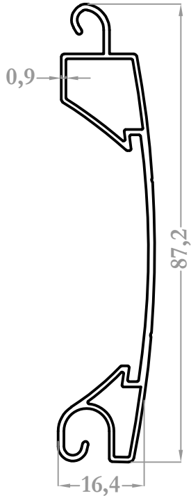
9231 0,538 kg/m
