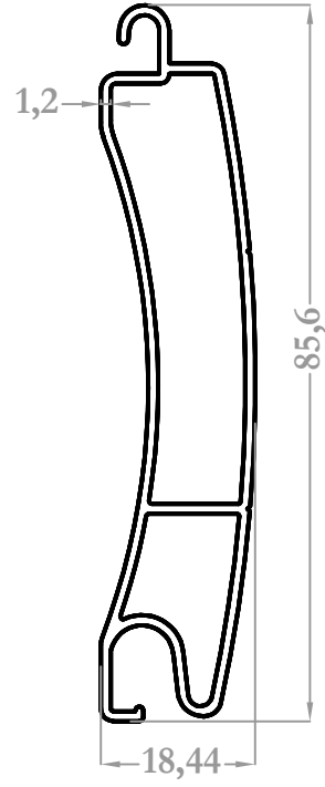
1703 0,705 kg/m
