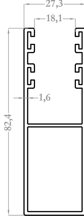
9489 1,073 kg/m
