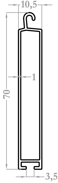
9230 0,440 kg/m
