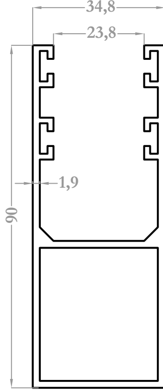
9127 1,452 kg/m
