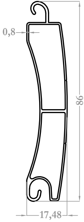
1705 0,536 kg/m
