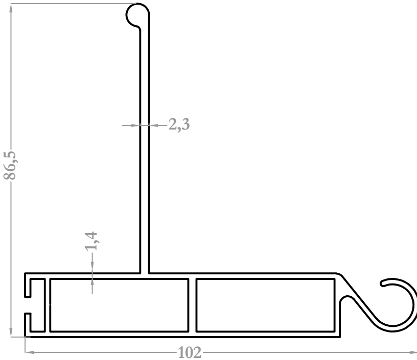
9580 1,490 kg/m
