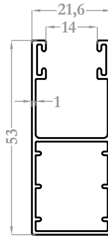
37008 0,460 kg/m
