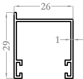
0002 0,254 kg/m
