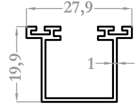
8847 0,244 kg/m
