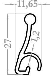
37015 0,222 kg/m
