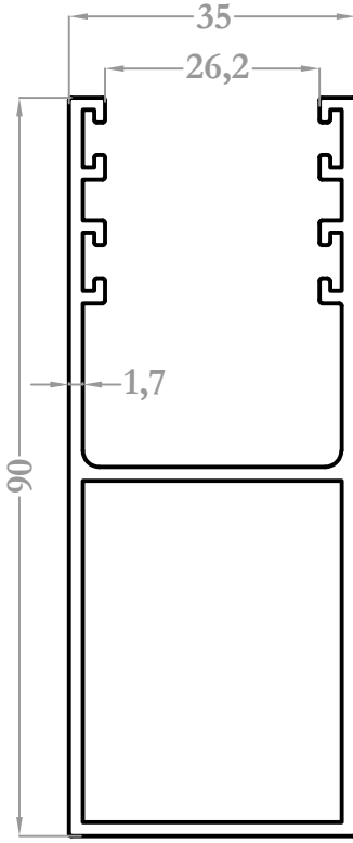
37005 1,252 kg/m
