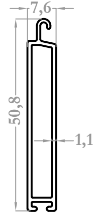
37013 0,328 kg/m
