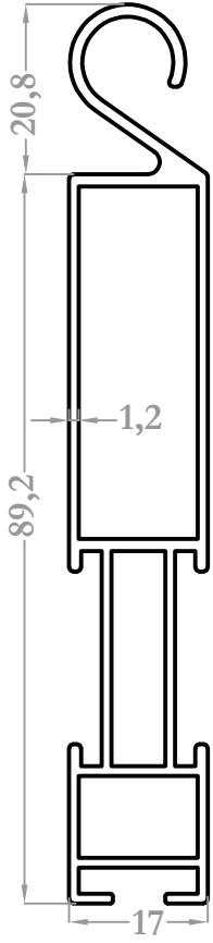
37009 1,056 kg/m
