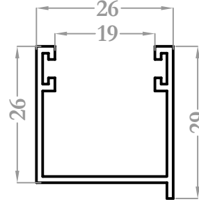
37021 0,304 kg/m
