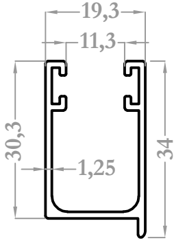
37019 0,342 kg/m
