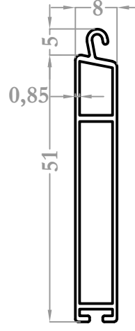
37012 0,327 kg/m
