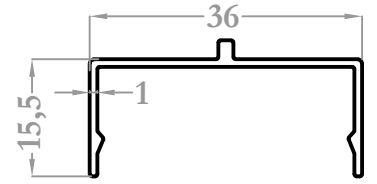
37018 0,197 kg/m
