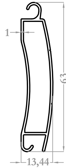
1702 0,400 kg/m
