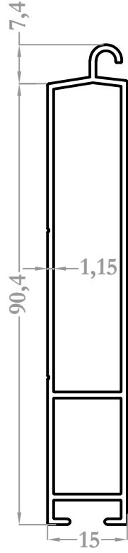
37010 0,691 kg/m
