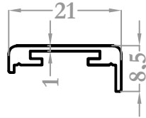
8142 0,141 kg/m
