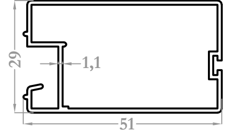
2118 0,536 kg/m
