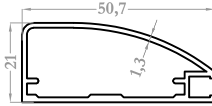
8094 0,520 kg/m
