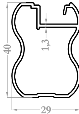
2112 0,482 kg/m
