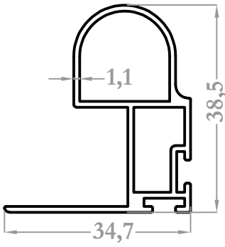
8940 0,459 kg/m
