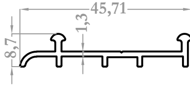
8402 0,258 kg/m
