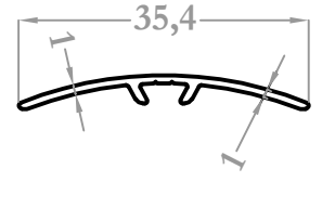
8937 0,113 kg/m
