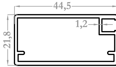
8103 0,561 kg/m
