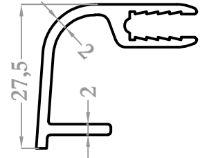
9307 0,434 kg/m
