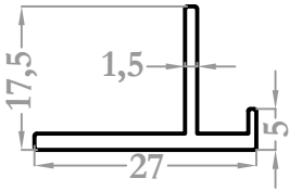
9076 0,217 kg/m
