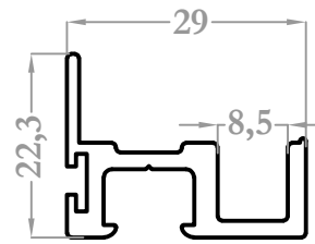
8354 0,436 kg/m
