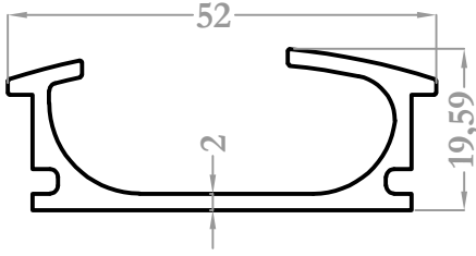
8351 0,633 kg/m
