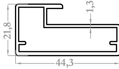
8164 0,544 kg/m
