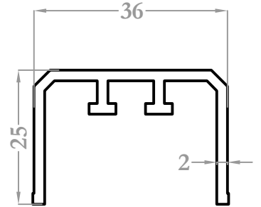
8161 0,529 kg/m
