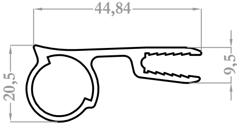
8962 0,557 kg/m
