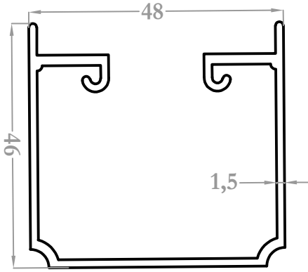
2126 0,772 kg/m
