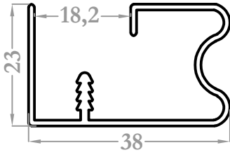
8167 0,369 kg/m
