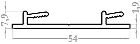
5022 0,419 kg/m
