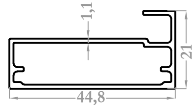
9041 0,412 kg/m
