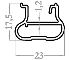
2110 0,256 kg/m
