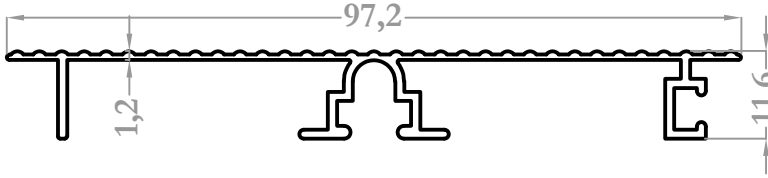
8089 0,469 kg/m
