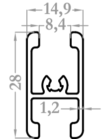
8290 0,350 kg/m
