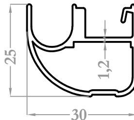
2111 0,420 kg/m
