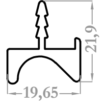
8842 0,360 kg/m
