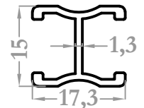
2108 0,182 kg/m
