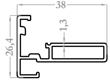
8228 0,435 kg/m
