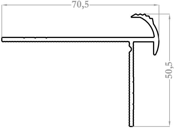
9249 0,660 kg/m
