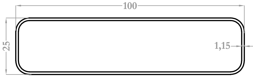
819 0,735 kg/m
