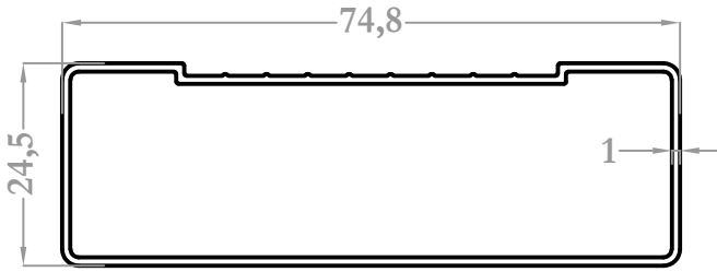
9590 0,531 kg/m
