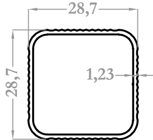
8789 0,310 kg/m
