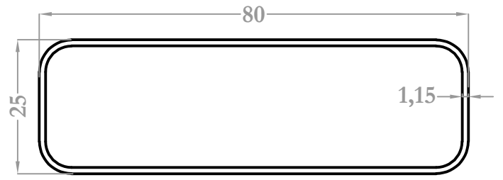
820 0,610 kg/m
