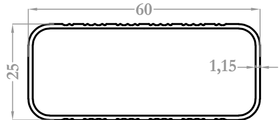
9635 0,458 kg/m
