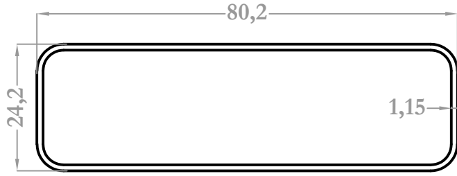
811 0,612 kg/m
