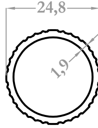
9087 0,337 kg/m
