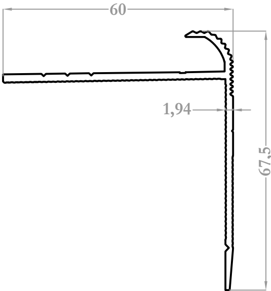
9247 0,655 kg/m
