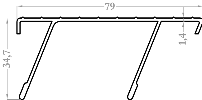
9605 0,630 kg/m
