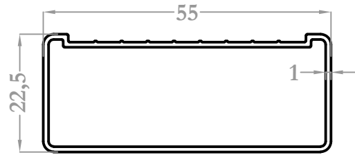
9591 0,412 kg/m
