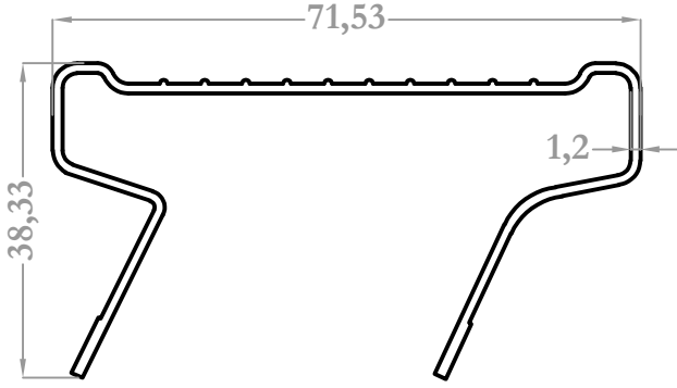
9037 0,630 kg/m
