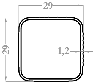
8197 0,285 kg/m
