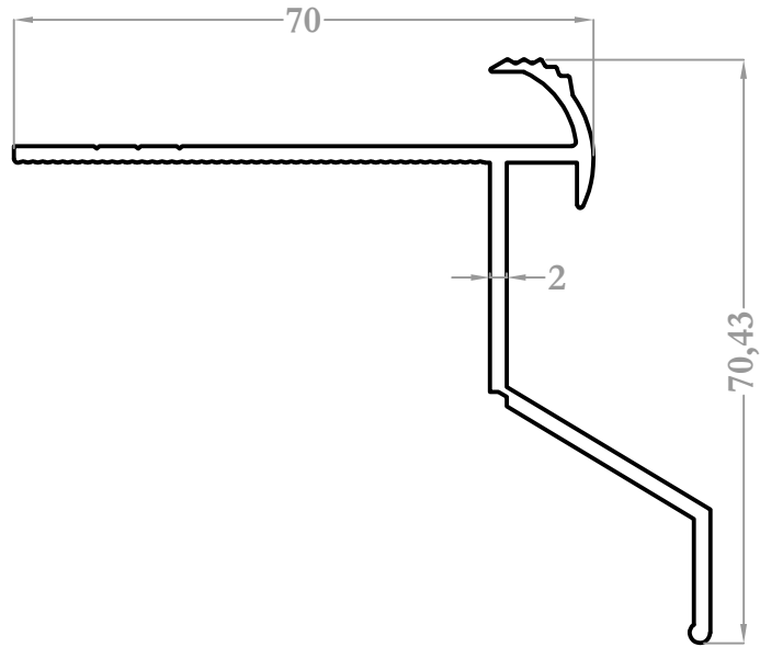
9248 0,851 kg/m
