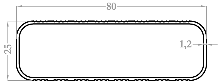
9026 0,580 kg/m
