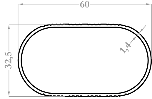
9088 0,547 kg/m
