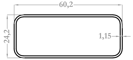
812 0,487 kg/m
