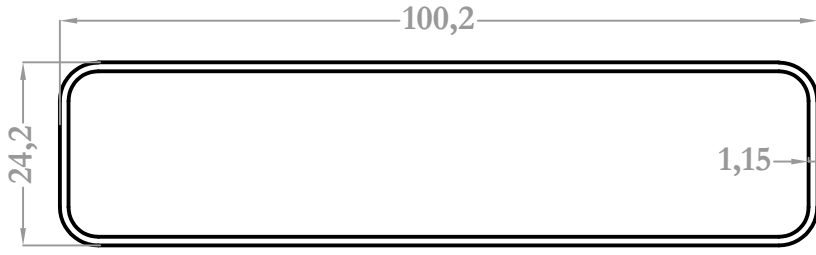
810 0,736 kg/m
