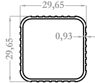
821 0,300 kg/m
