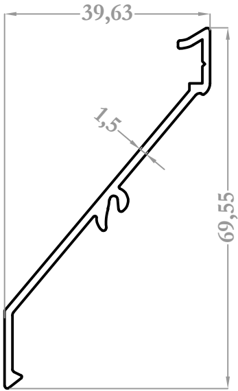
37117 0,422 kg/m
