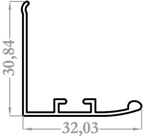
8113 0,240 kg/m
