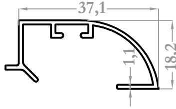
8912 0,263 kg/m
