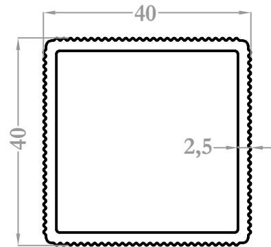
9258 0,898 kg/m
