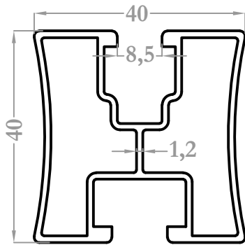
8904 0,817 kg/m
