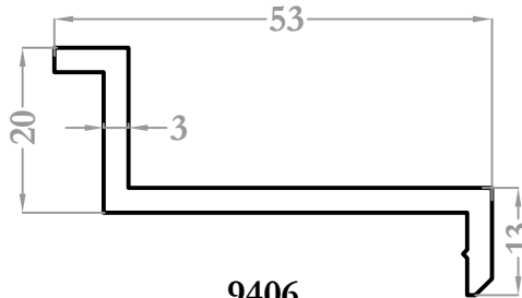
9406 0,646 kg/m
