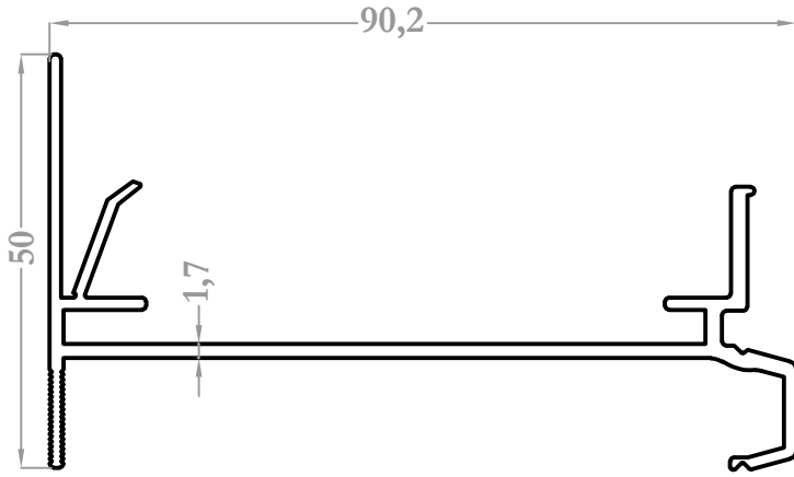
8721 0,916 kg/m
