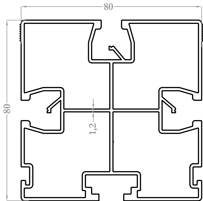
9576 2,465 kg/m
