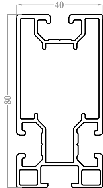
8831 1,712 kg/m
