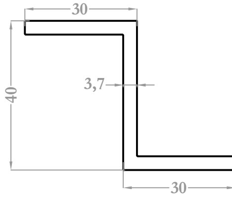
9368 0,928 kg/m
