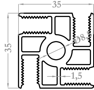
9192 1,206 kg/m
