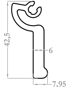
9191 0,789 kg/m
