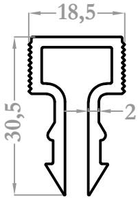
9549 0,477 kg/m
