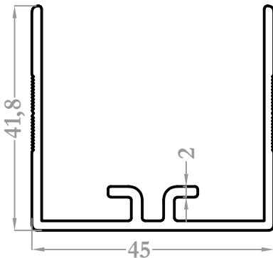
9189 0,705 kg/m
