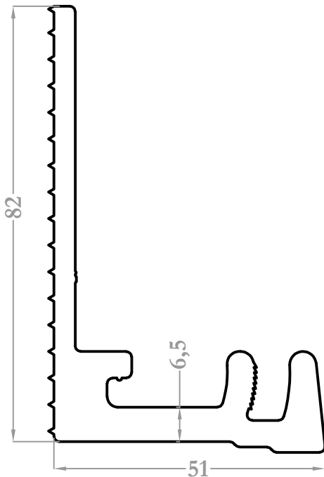
9608 2,289 kg/m
