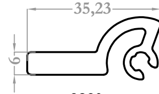
9280 0,631 kg/m
