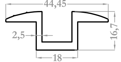
9184 0,581 kg/m
