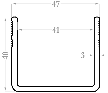
9551 0,947 kg/m
