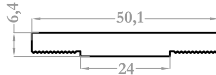
9456 0,786 kg/m
