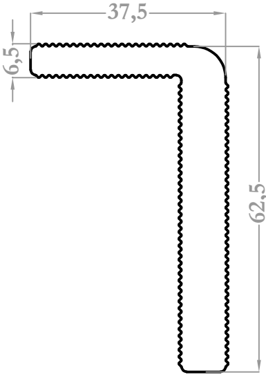
9259 1,960 kg/m
