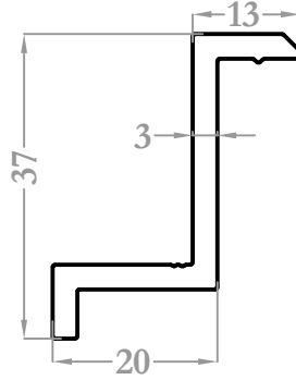
9428 0,515 kg/m
