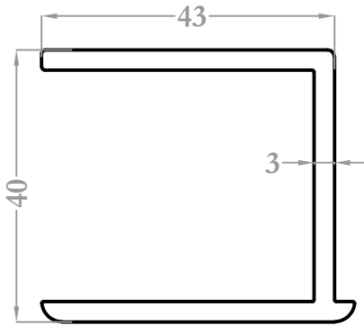
9256 0,989 kg/m
