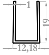
5032 0,130 kg/m
