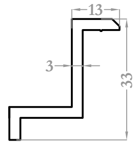
9532 0,482 kg/m
