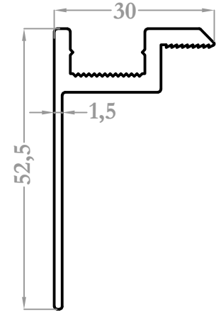
9194 0,561 kg/m
