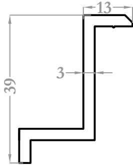
9534 0,531 kg/m
