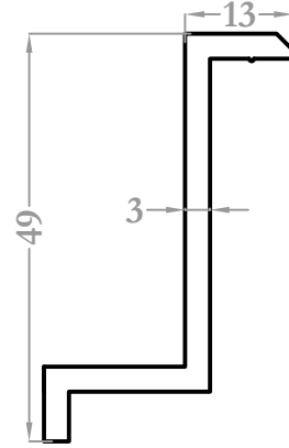
9539 0,612 kg/m
