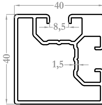
9477 0,886 kg/m
