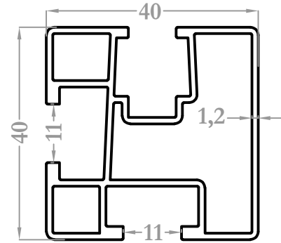
9545 0,840 kg/m
