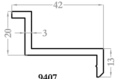
9407 0,556 kg/m
