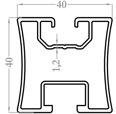
8834 0,802 kg/m
