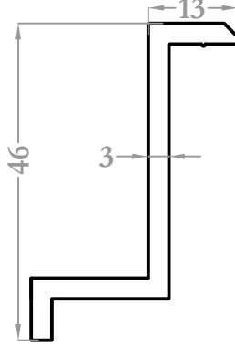
9538 0,588 kg/m
