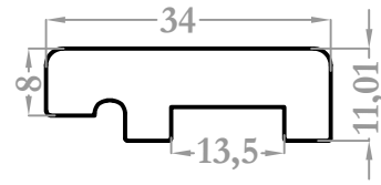
9350 0,771 kg/m
