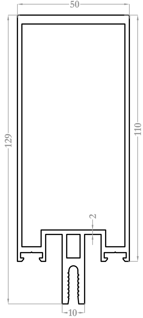
3213 2,566 kg/m
