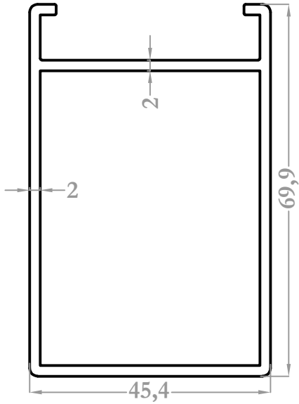
8603 1,233 kg/m
