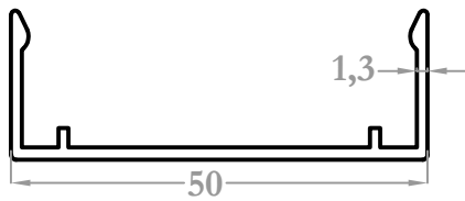
3224 0,343 kg/m
