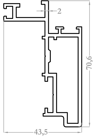
3095 1,178 kg/m
