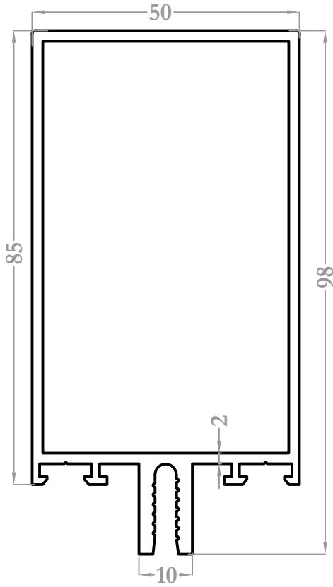
3214 1,730 kg/m
