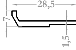
3218 0,172 kg/m
