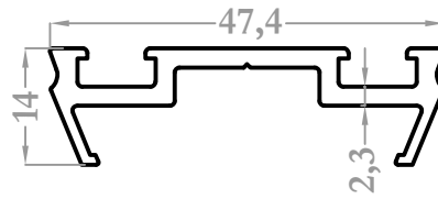
3226 0,494 kg/m
