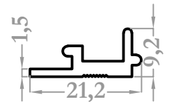
1721 0,196 kg/m
