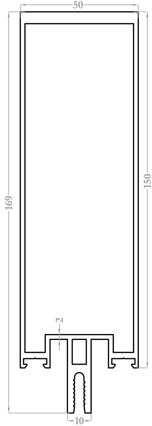
3219 3,125 kg/m
