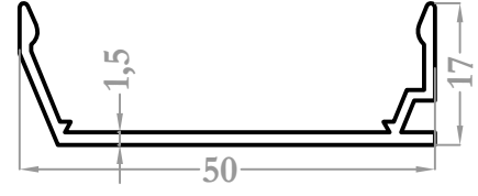
3222 0,319 kg/m
