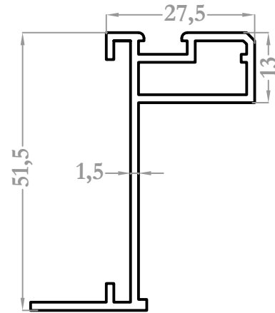
3216 0,577 kg/m
