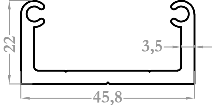
3217 0,780 kg/m
