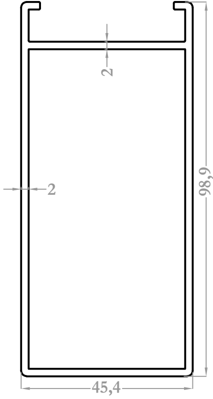
8604 1,547 kg/m
