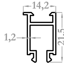
3027 0,210 kg/m
