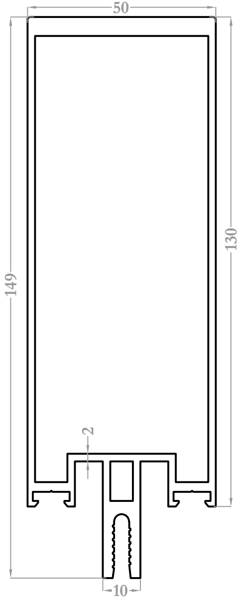
3603 2,905 kg/m
