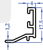
E3610 1411 0,130 kg/m
