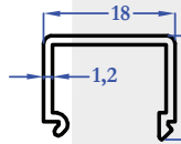
E 3609 0,150 kg/m
