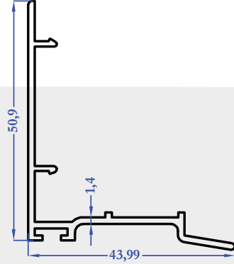
E 2900 1416 0,425 kg/m
