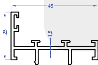
1417 0,454 kg/m
