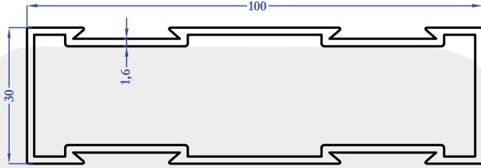
1413 1,259 kg/m
