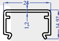
1419 0,195 kg/m
