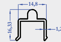
E3607 1406 0,179 kg/m
