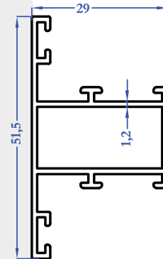
E3601 1409 0,518 kg/m
