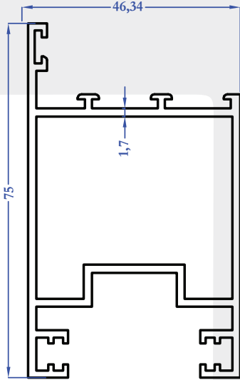
1414 1,278 kg/m
