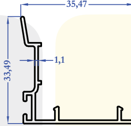
E 3604 1407 0,261 kg/m
