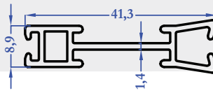
8705 0,342 kg/m
