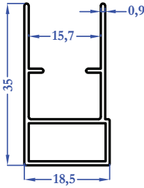
M5743 0,267 kg/m
