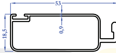
M5274 0,405 kg/m
