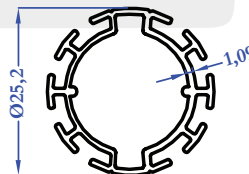
M5171 0,311 kg/m
