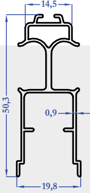
M5744 0,380 kg/m
