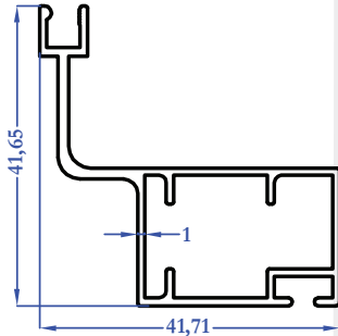
R9246 0,475 kg/m
