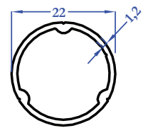
R9087 0,233 kg/m
