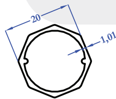
M5658 0,216 kg/m
