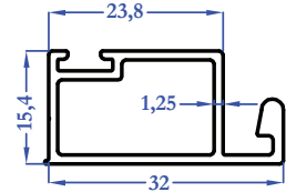
M5754 0,347 kg/m
