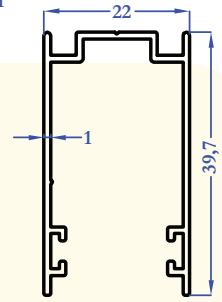
8706 0,323 kg/m
