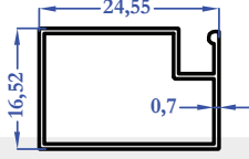
M5095 0,164 kg/m
