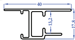
M5091 0,310 kg/m
