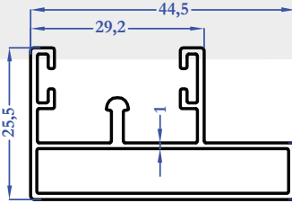
M5520 0,485 kg/m
