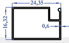
M6200 0,139 kg/m
