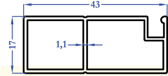
M5491 0,402 kg/m
