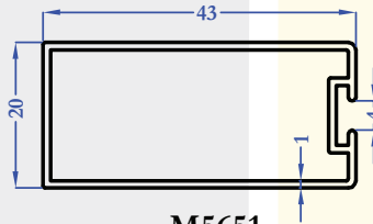
M5651 0,355 kg/m
