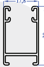
M5090 0,247 kg/m
