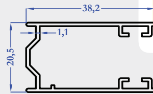
M5239 0,336 kg/m
