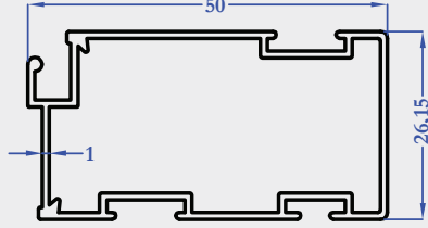
M5652 0,498 kg/m
