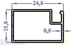
M6129 0,184 kg/m
