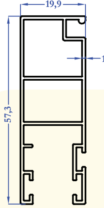
M5076 0,554 kg/m
