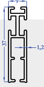
M5547 0,325 kg/m
