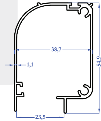
8708 0,562 kg/m
