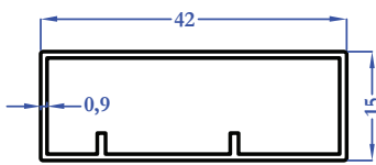
R9237 0,286 kg/m
