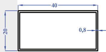
M5021 0,252 kg/m
