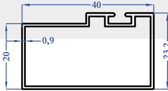
M5655 0,331 kg/m
