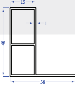
M5654 0,385 kg/m
