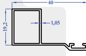
M5273 0,265 kg/m
