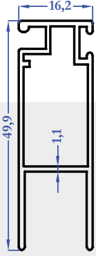
E1774 0,450 kg/m
