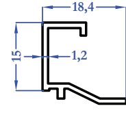
M5659 0,151 kg/m
