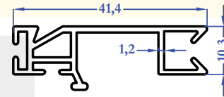
M5157 0,360 kg/m
