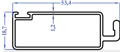
E1775 0,522 kg/m
