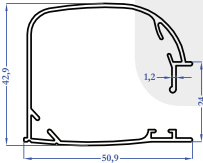
M5439 0,543 kg/m
