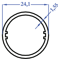
E1431 0,308 kg/m
