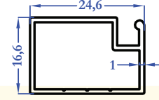
M6128 0,230 kg/m
