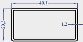
E1776 0,375 kg/m
