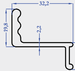
M5662 0,454 kg/m
