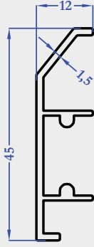
E1590 0,312 kg/m
