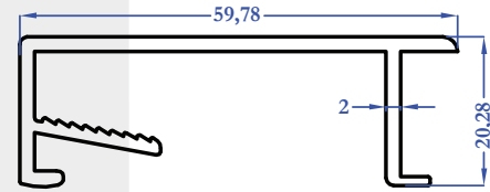
M5124 0,649 kg/m
