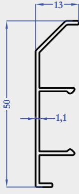
M5445 0,248 kg/m
