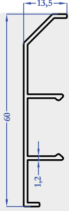
M5020 0,497 kg/m
