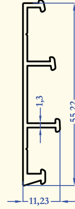
M5323 0,347 kg/m
