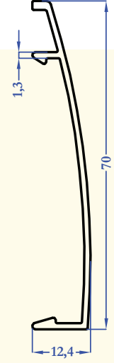
M5324 0,335 kg/m
