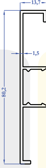
E1557 0,510 kg/m
