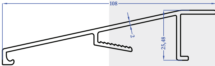
M5123 0,932 kg/m
