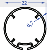
M6036 0,156 kg/m
