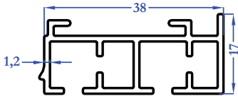
9396 0,424 kg/m
