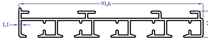
M6010 0,737 kg/m
