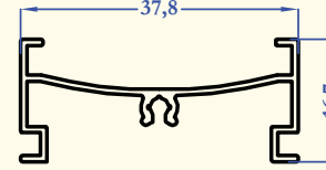
9377 M5098 0,210 kg/m
