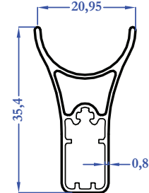
M5790 0,285 kg/m
