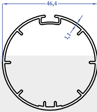
M5785 0,521 kg/m
