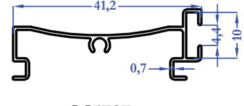
M5787 0,180 kg/m
