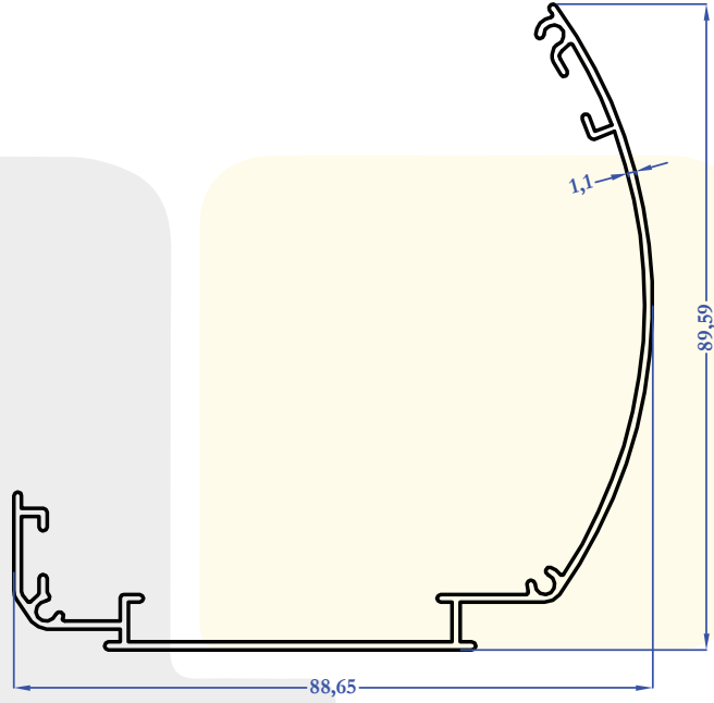
M6021 0,690 kg/m
