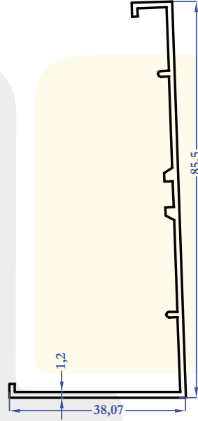
9459 0,471 kg/m
