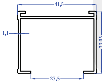
9440 0,392 kg/m
