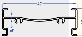
9379 M5516 0,240 kg/m
