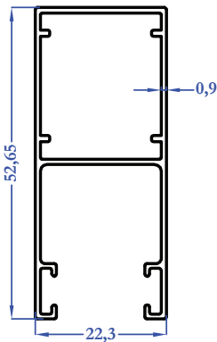
M5667 0,413 kg/m
