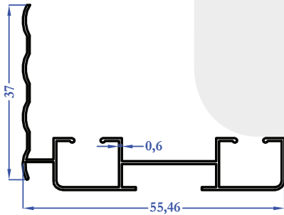
M5937 0,254 kg/m
