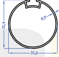
8824 0,262 kg/m
