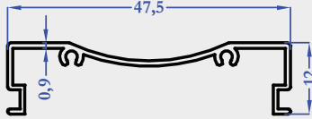
9376 E2722 0,225 kg/m
