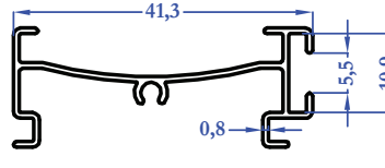
M5888 0,223 kg/m
