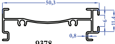
9378 M5789 0,245 kg/m
