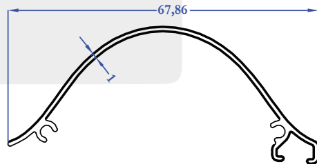
M5932 0,310 kg/m
