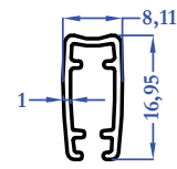
M5684 0,126 kg/m
