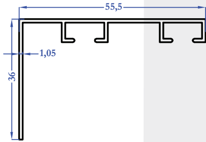
M5862 0,355 kg/m
