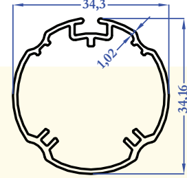
9205 0,369 kg/m
