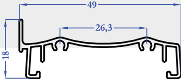
M5189 0,290 kg/m
