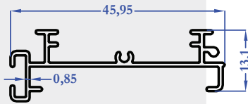
M5666 0,223 kg/m
