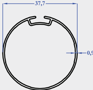
M5784 0,291 kg/m
