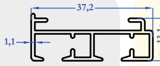
M6012 0,319 kg/m
