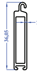
M5668 0,249 kg/m
