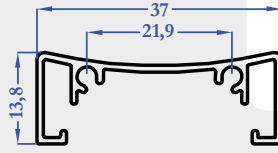
M5188 0,248 kg/m
