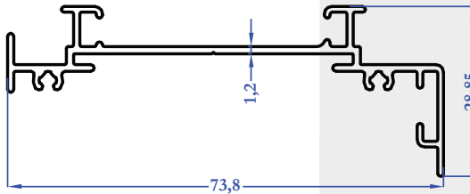
M5800 0,497 kg/m
