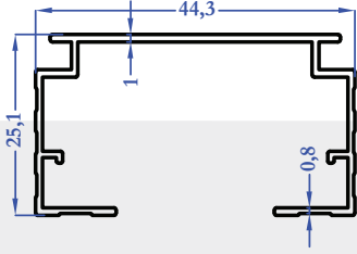
8826 0,319 kg/m
