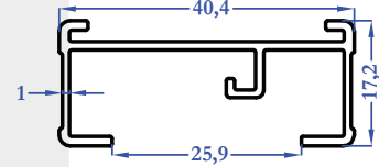
9481 0,309 kg/m
