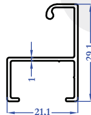
M5671 0,214 kg/m
