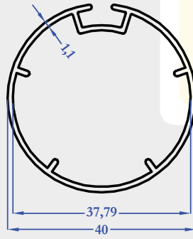
M5369 0,435 kg/m
