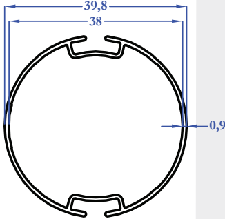
M5915 0,332 kg/m
