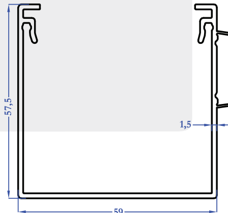
M6037 0,819 kg/m
