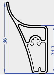
M6014 0,104 kg/m
