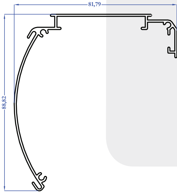
M5938 0,694 kg/m
