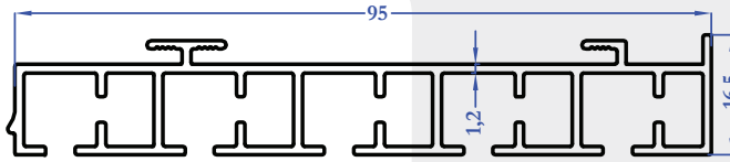
9399 0,935 kg/m
