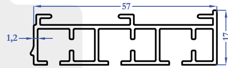
9397 0,604 kg/m
