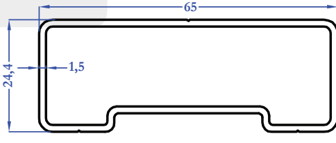
E3881 0,711 kg/m
