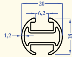
9400 0,280 kg/m
