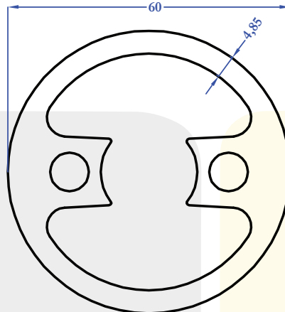
1812 3,336 kg/m
