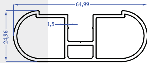
M5950 0,853 kg/m
