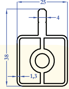
M5215 0,717 kg/m
