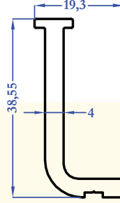
M5214 0,542 kg/m
