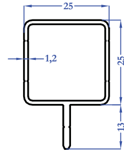
M5508 0,367 kg/m
