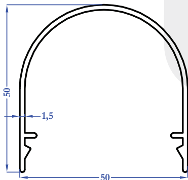
1803 0,556 kg/m
