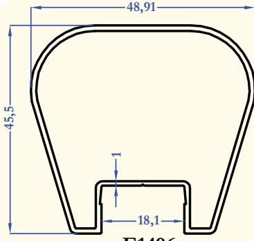
E1496 0,561 kg/m
