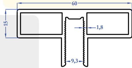
M5454 0,992 kg/m
