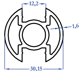
1818 0,662 kg/m
