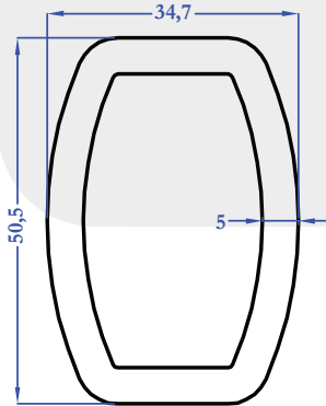
M5217 1,782 kg/m
