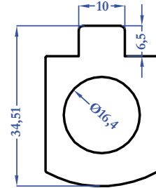
E2737 1,373 kg/m
