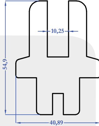
R9490 3,202 kg/m
