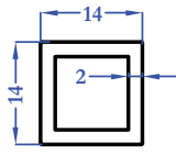
M5154 0,258 kg/m
