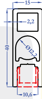
M5456 0,650 kg/m
