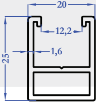
M5705 0,389 kg/m
