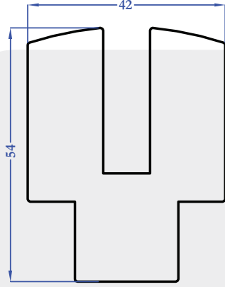
1810 4,129 kg/m
