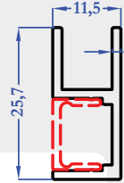
M5017 0,231 kg/m
