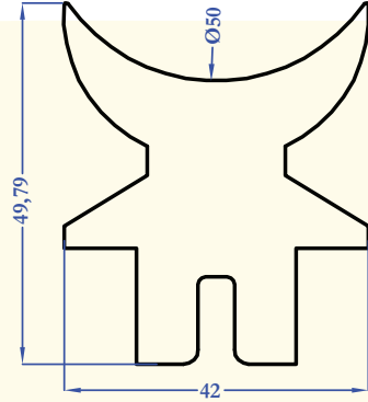
1817 3,010 kg/m
