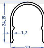
1801 0,196 kg/m
