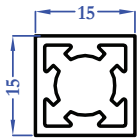
E3667 0,306 kg/m
