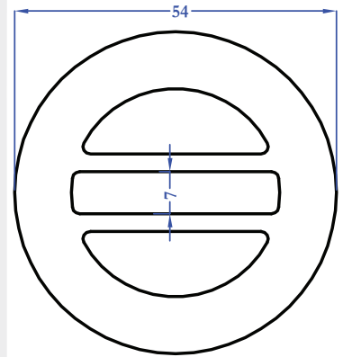
E2740 4,157 kg/m
