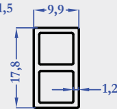
M5707 0,194 kg/m
