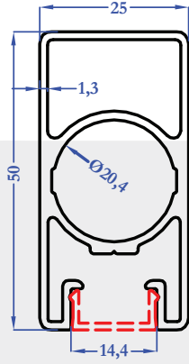
M5416 0,825 kg/m
