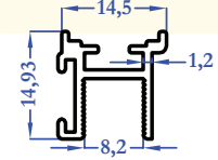
36923 0,169 kg/m
