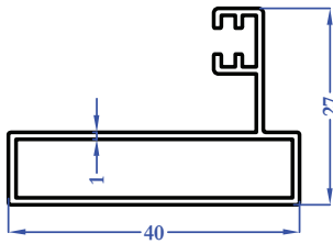
M5755 0,355 kg/m
