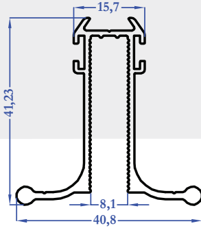
M5467 0,531 kg/m
