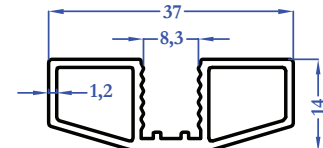
M5542 0,376 kg/m
