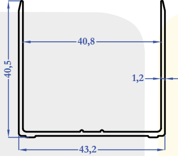
M5083 0,398 kg/m
