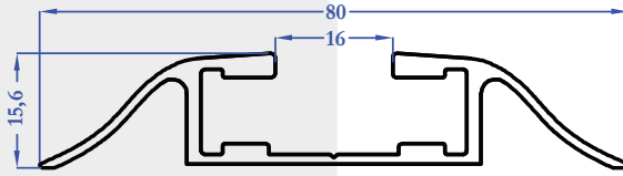
M5081 0,655 kg/m
