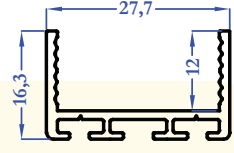
M5280 0,289 kg/m
