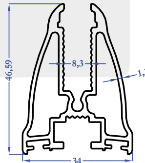
M5197 0,884 kg/m
