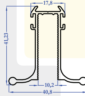
M5248 0,529 kg/m
