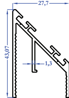
M5851 0,495 kg/m
