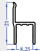
M5321 0,116 kg/m
