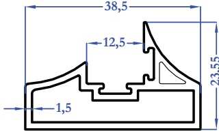
30161 0,545 kg/m
