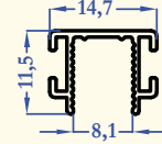
M5465 0,108 kg/m
