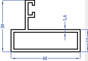
R9202 0,546 kg/m
