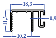
M5249 0,123 kg/m
