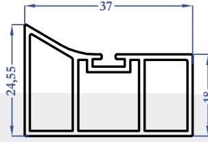
M5034 0,501 kg/m
