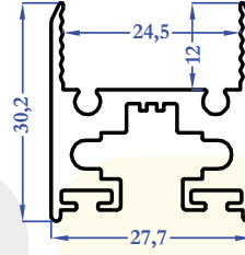
M5272 0,735 kg/m
