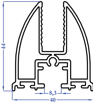
M5765 0,906 kg/m
