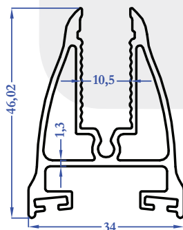
M5060 0,832 kg/m
