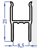
M5198 0,146 kg/m
