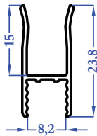
M5033 0,142 kg/m
