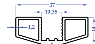
M5089 0,372 kg/m
