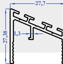
M5852 0,354 kg/m
