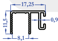
M5466 0,120 kg/m
