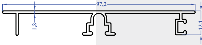
8270 0,536 kg/m
