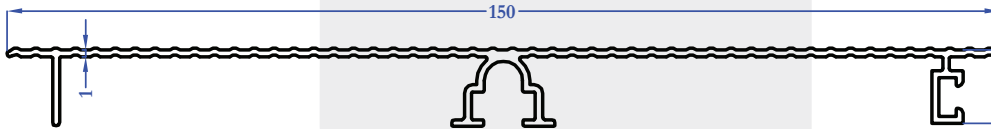
8272 0,598 kg/m
