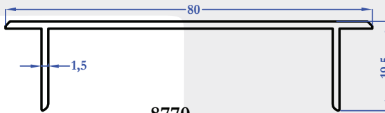
8770 0,466 kg/m
