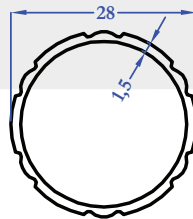
8418 0,310 kg/m
