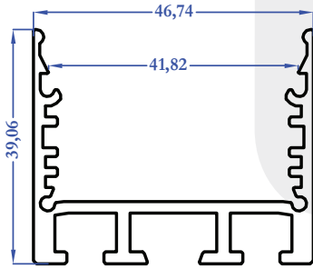
9511 0,916 kg/m
