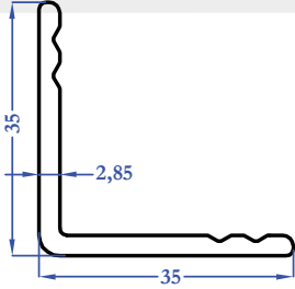
8817 0,492 kg/m
