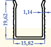
9040 0,152 kg/m
