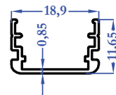
M5190 0,124 kg/m
