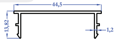
8697 0,233 kg/m
