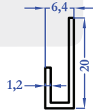
9558 0,107 kg/m
