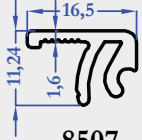
8507 0,181 kg/m
