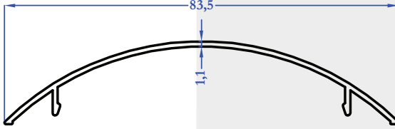
8655 0,310 kg/m
