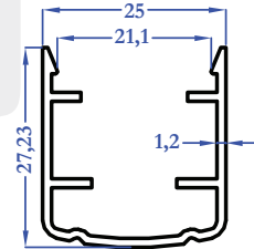
8703 0,306 kg/m
