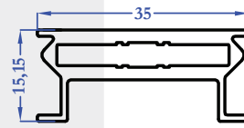
M5478 0,480 kg/m
