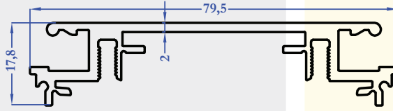
8506 0,902 kg/m
